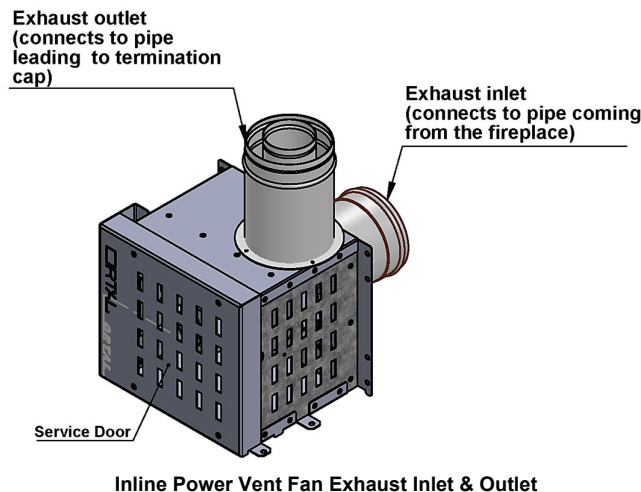
Inline Power Vent Fan Exhaust Inlet & Outlet
