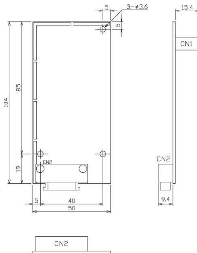
図 1.2-1 インタフェースカード外形
