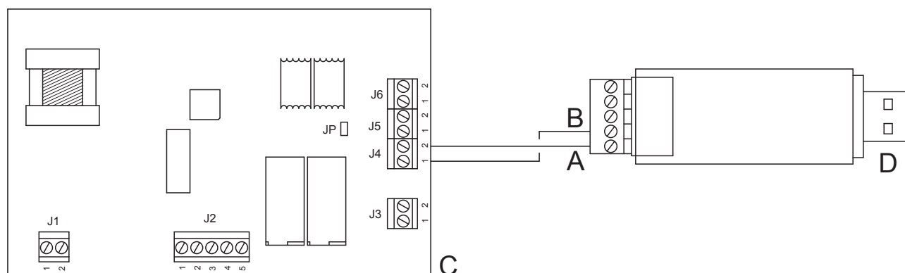
Figura 4.6 Collegamento convertitore USB/RS485
