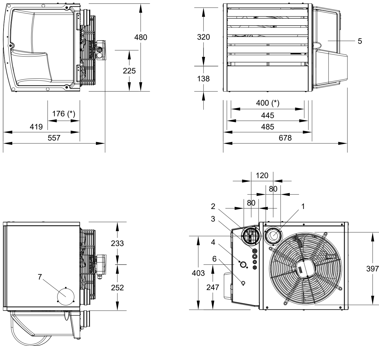
Figura 1.1 Dimensioni unità
