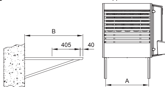
Figura 2.4 Installazione con mensola di supporto
