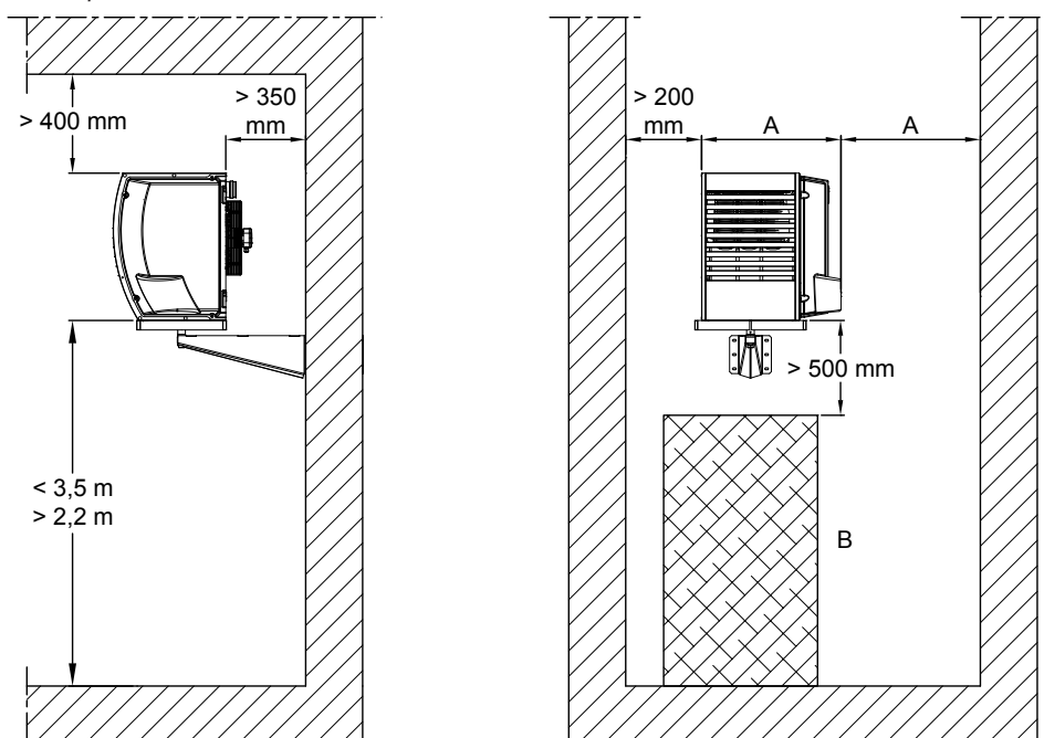
Figura 2.2 Distanze di rispetto
