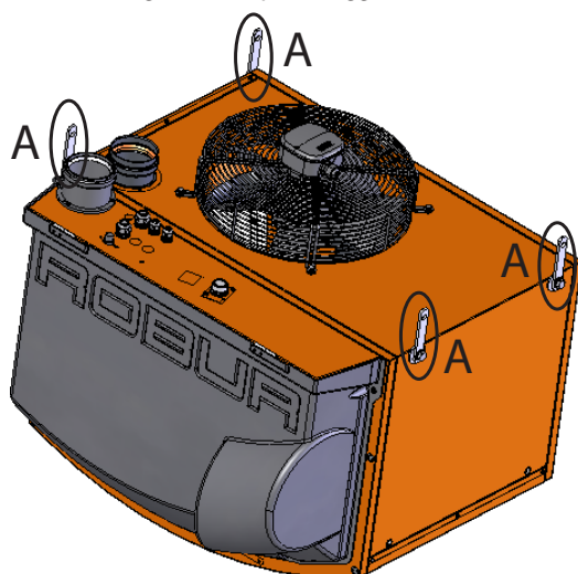
Figura 2.5 Staffe generatore per fissaggio a soffitto
