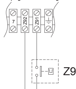
Figura 4.7 Collegamento consenso esterno per la gestione dell'accensione/spegnimento del generatore
