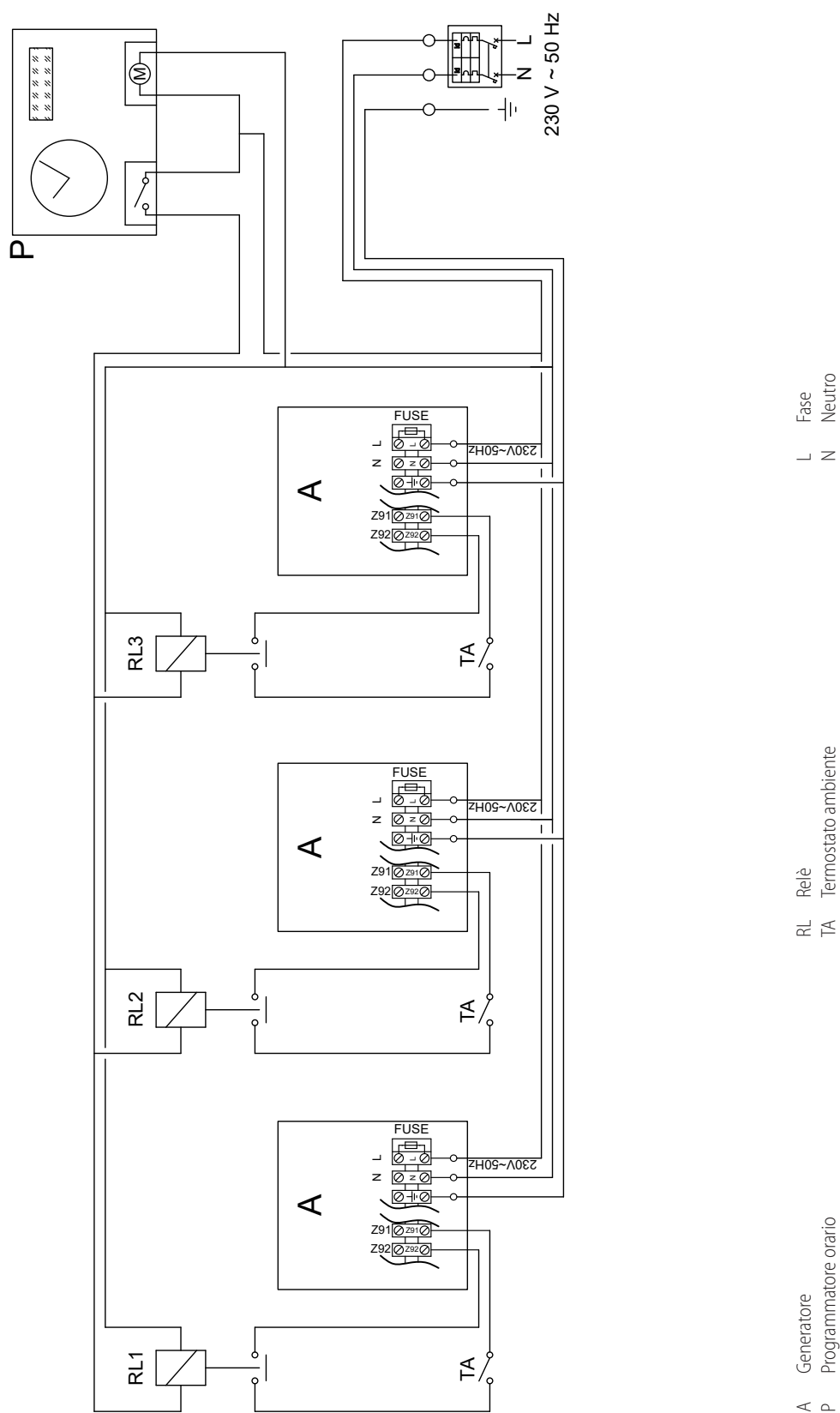
Figura 4.11 Schema di collegamento di più apparecchi con un orologio programmatore e più termostati ambiente
