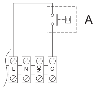
Figura 4.9 Collegamento selettore del livello di potenza del generatore
