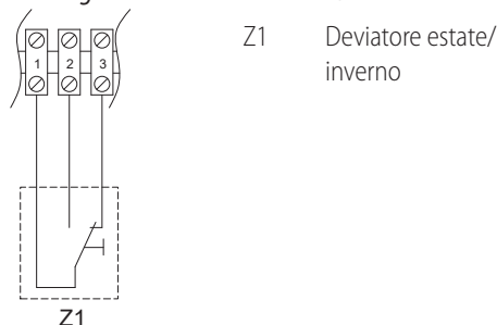
Figura 4.8 Collegamento deviatore estate/inverno
