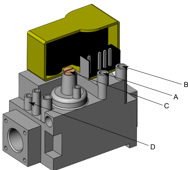
Figura 5.1 Valvola gas
