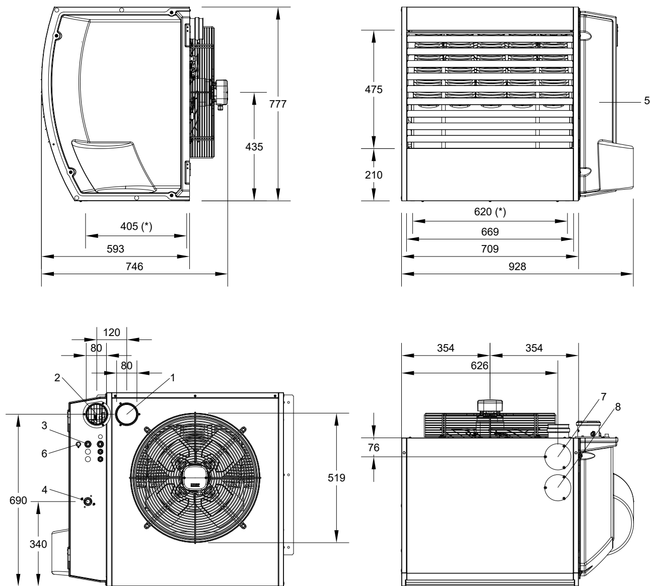
Figura 1.4 Dimensioni unità
