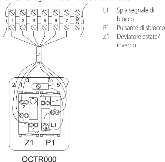
Figura 4.3 Collegamento comando base a 2 tasti
