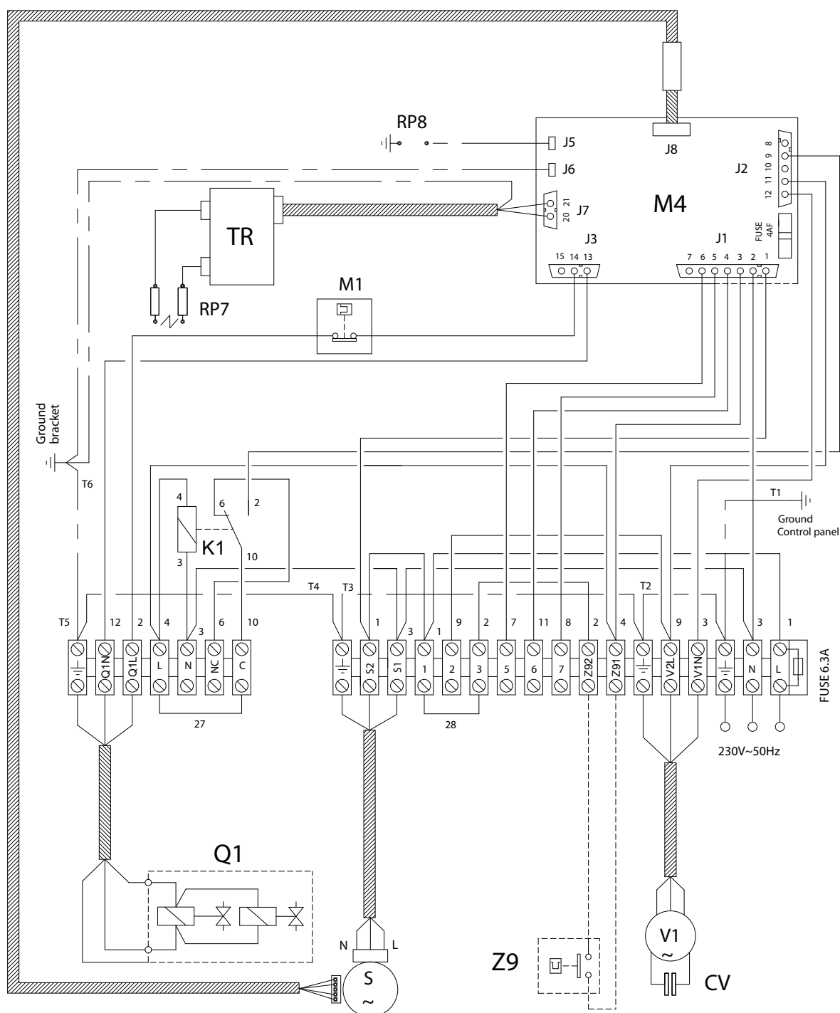
Figura 1.14 Schema elettrico
