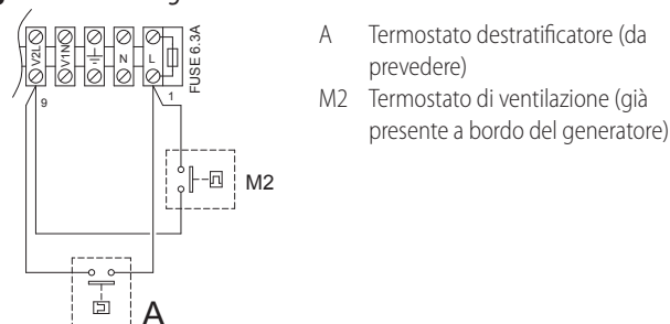
Figura 4.10 Collegamento termostato destratificatore
