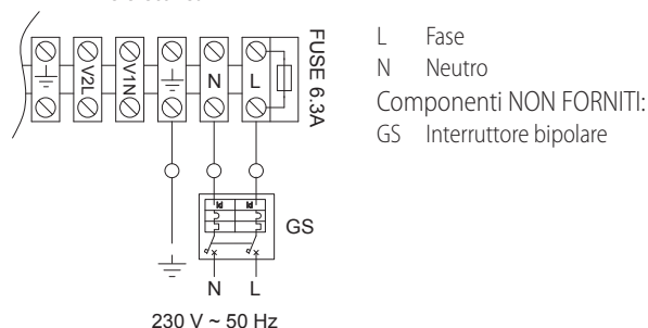
Figura 4.1 Collegamento dell'apparecchio alla rete di alimentazione elettrica
