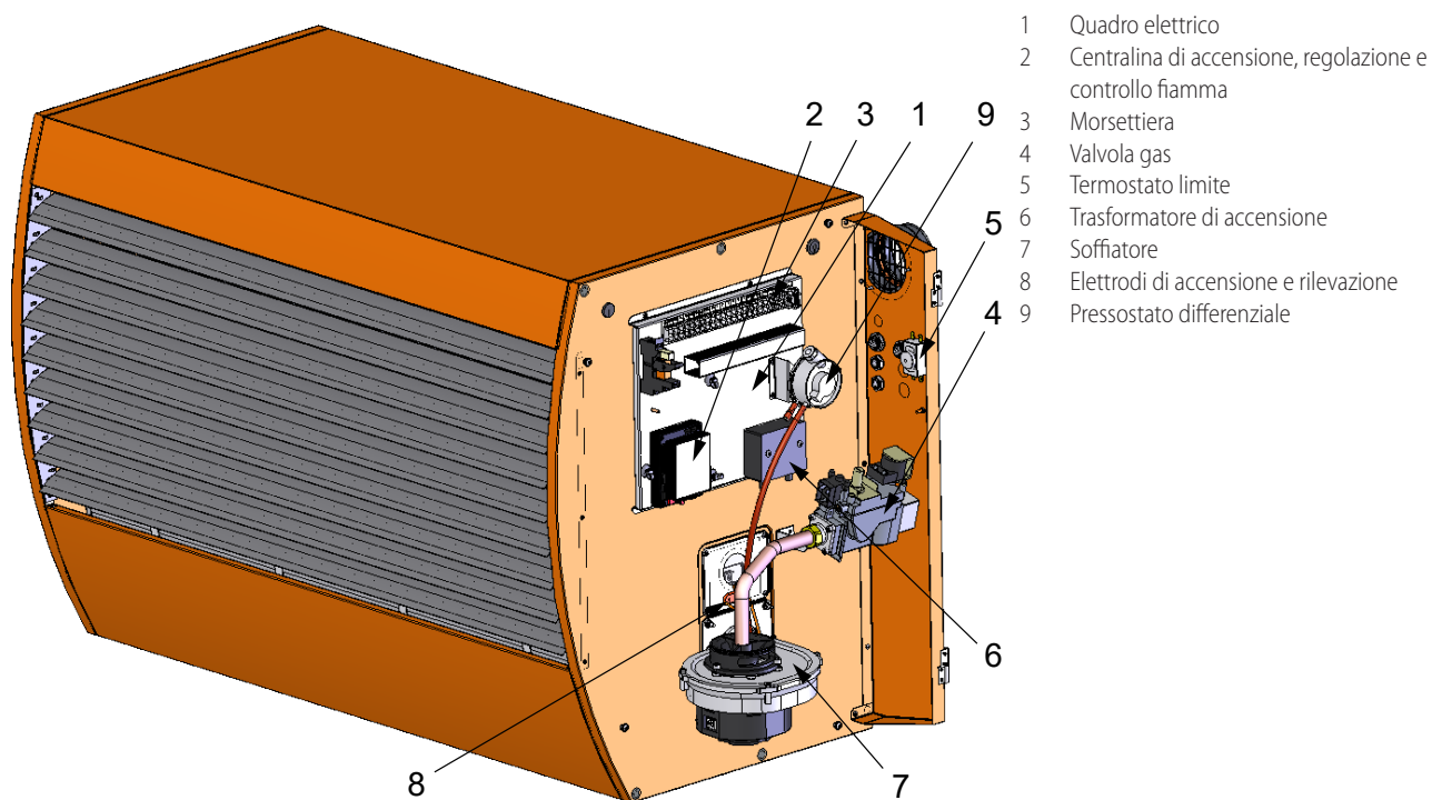
Figura 1.13 Componenti interni
