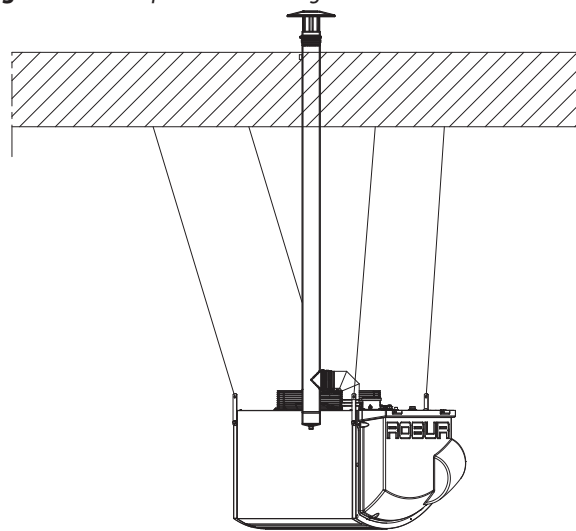
Figura 3.9 Esempio installazione generatore a lancio verticale
