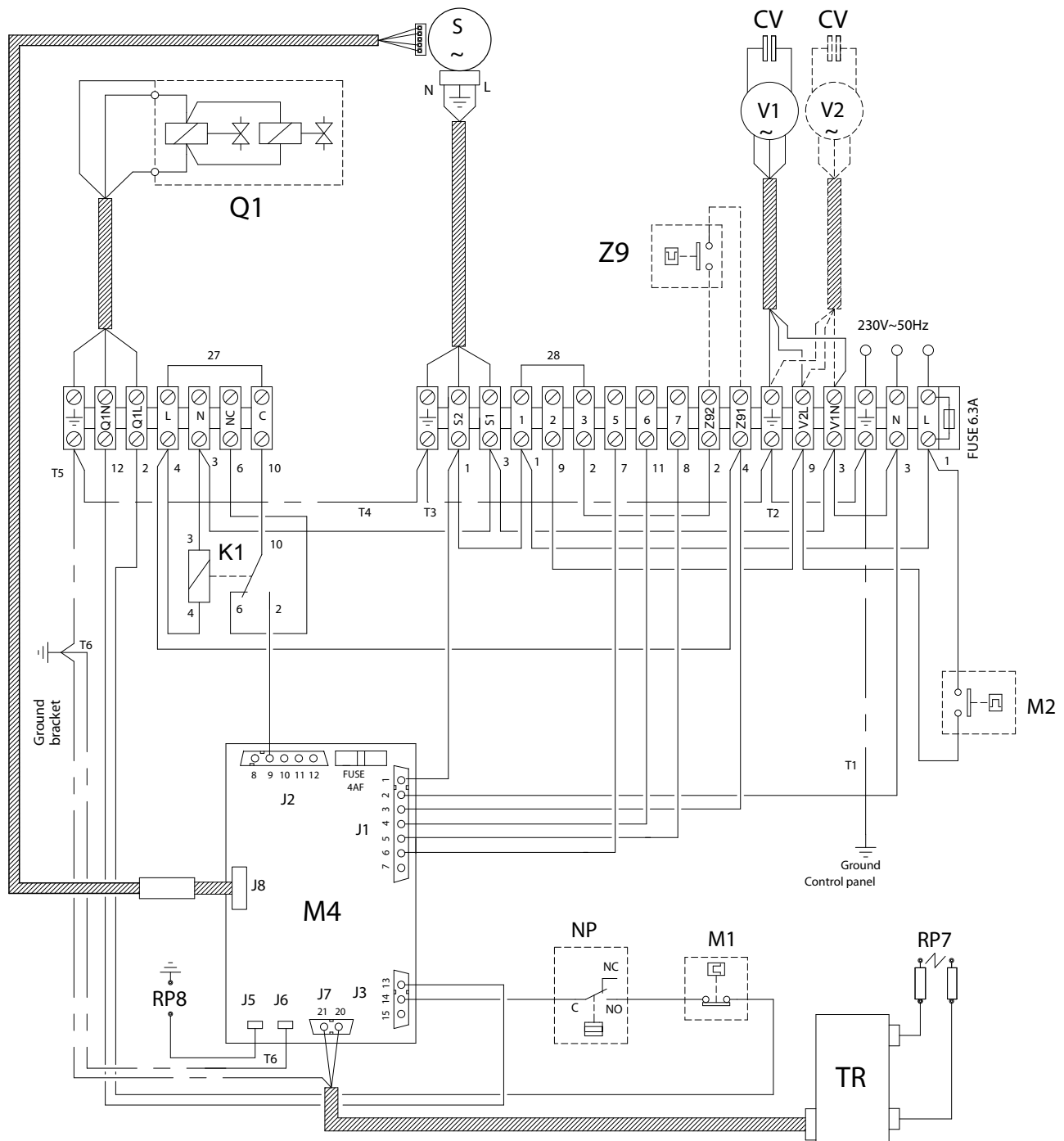
Figura 1.15 Schema elettrico
