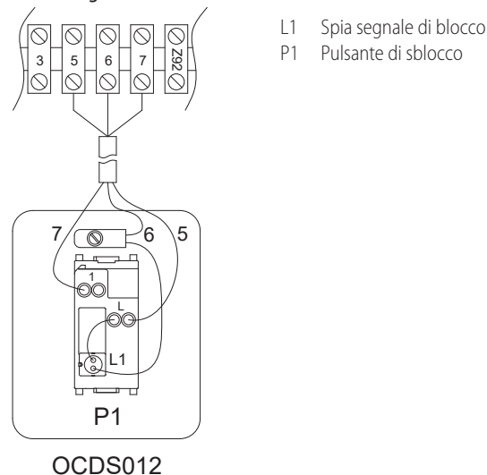
Figura 4.2 Collegamento comando base a 1 tasto
