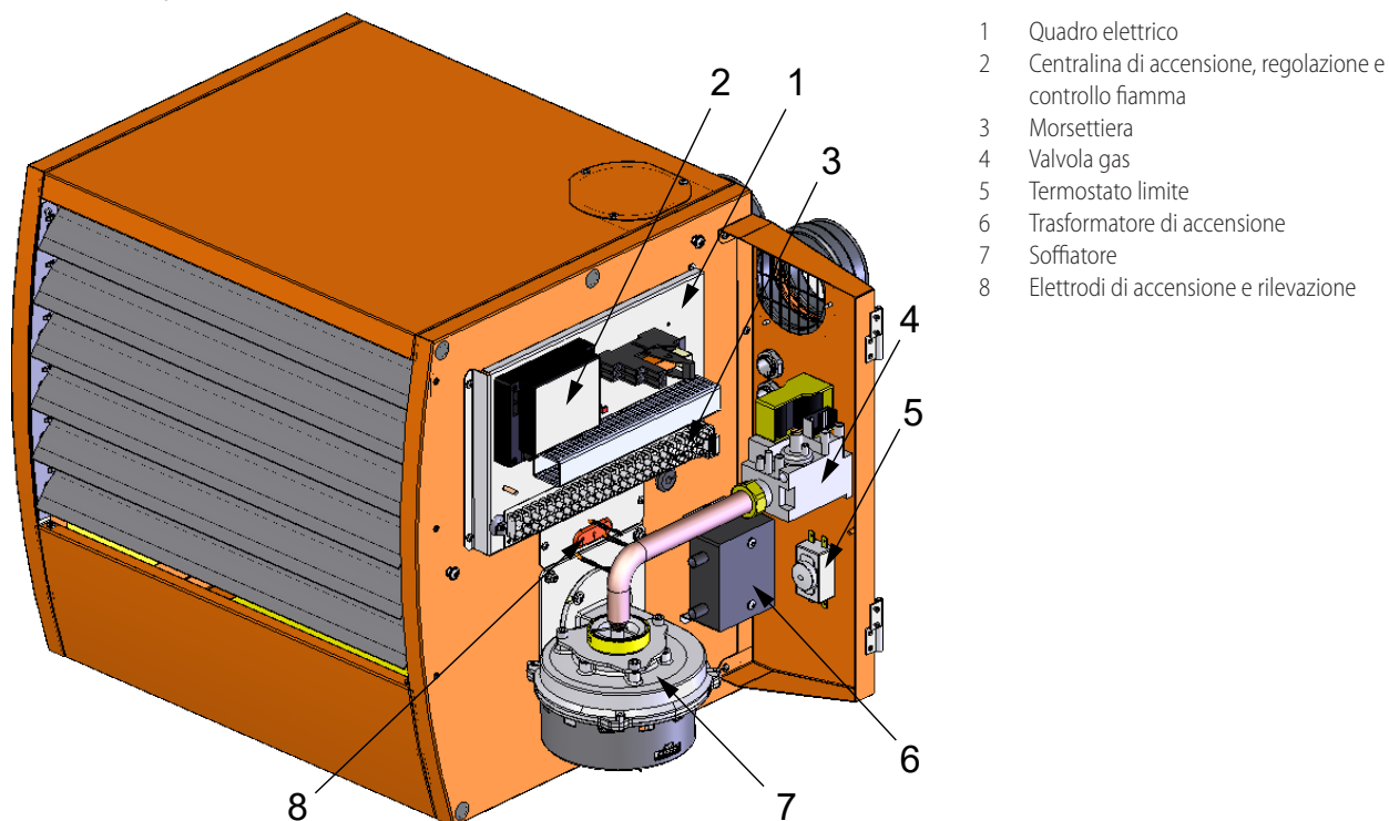
Figura 1.12 Componenti interni
