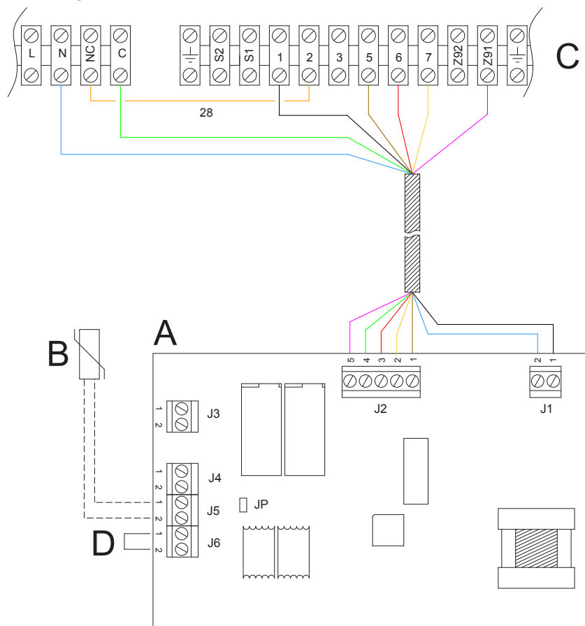
Figura 4.4 Collegamento termoregolatore OTRG005
