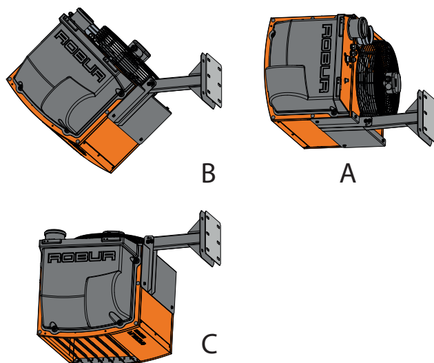
Figura 2.6 Posizioni staffa OSTF020
