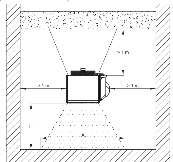
Figura 2.3 Distanze di rispetto
