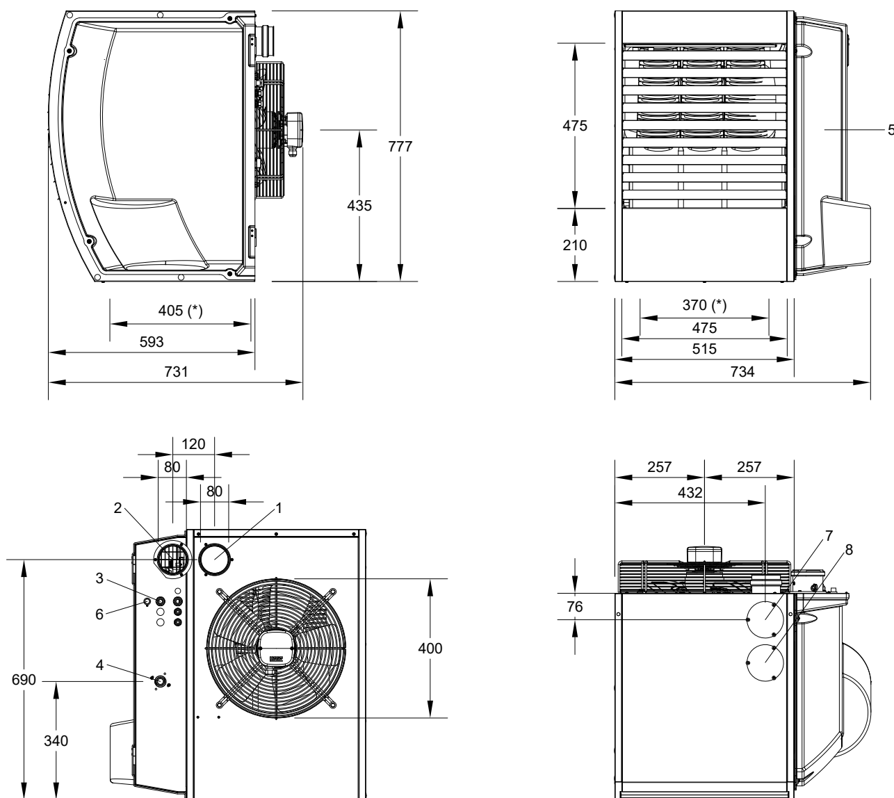
Figura 1.3 Dimensioni unità
