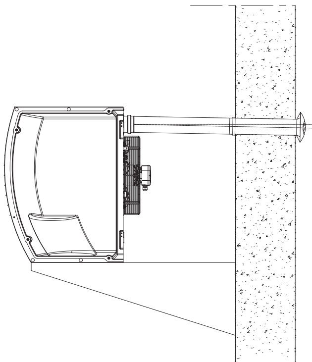
Figura 3.7 Pendenza tubi orizzontali
