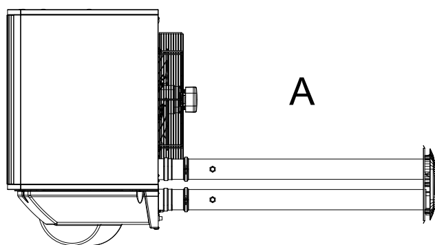
Figura 3.3 Installazione tipo C13 con tubi separati Ø 80
