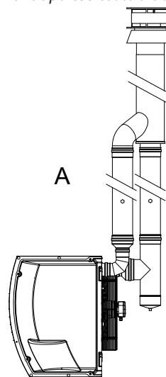
Figura 3.5 Installazione tipo C33 coassiale a tetto
