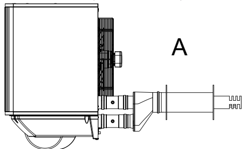
Figura 3.4 Installazione tipo C13 coassiale a parete con tubi Ø 80
