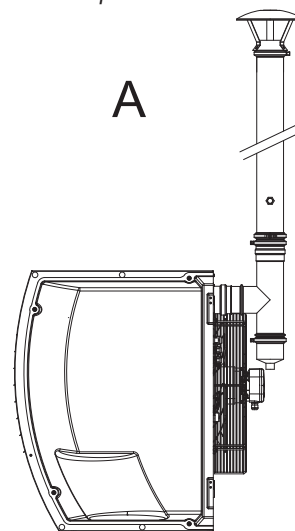
Figura 3.2 Installazione tipo B23 con tubo fumi a tetto Ø 80
