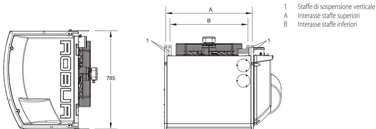
Figura 1.11 Posizione staffe generatori a lancio verticale
