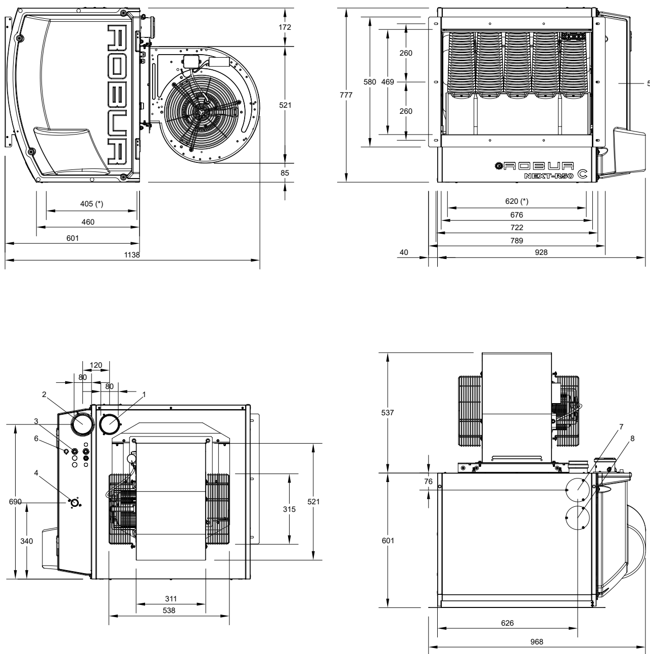
Figura 1.9 Dimensioni unità
