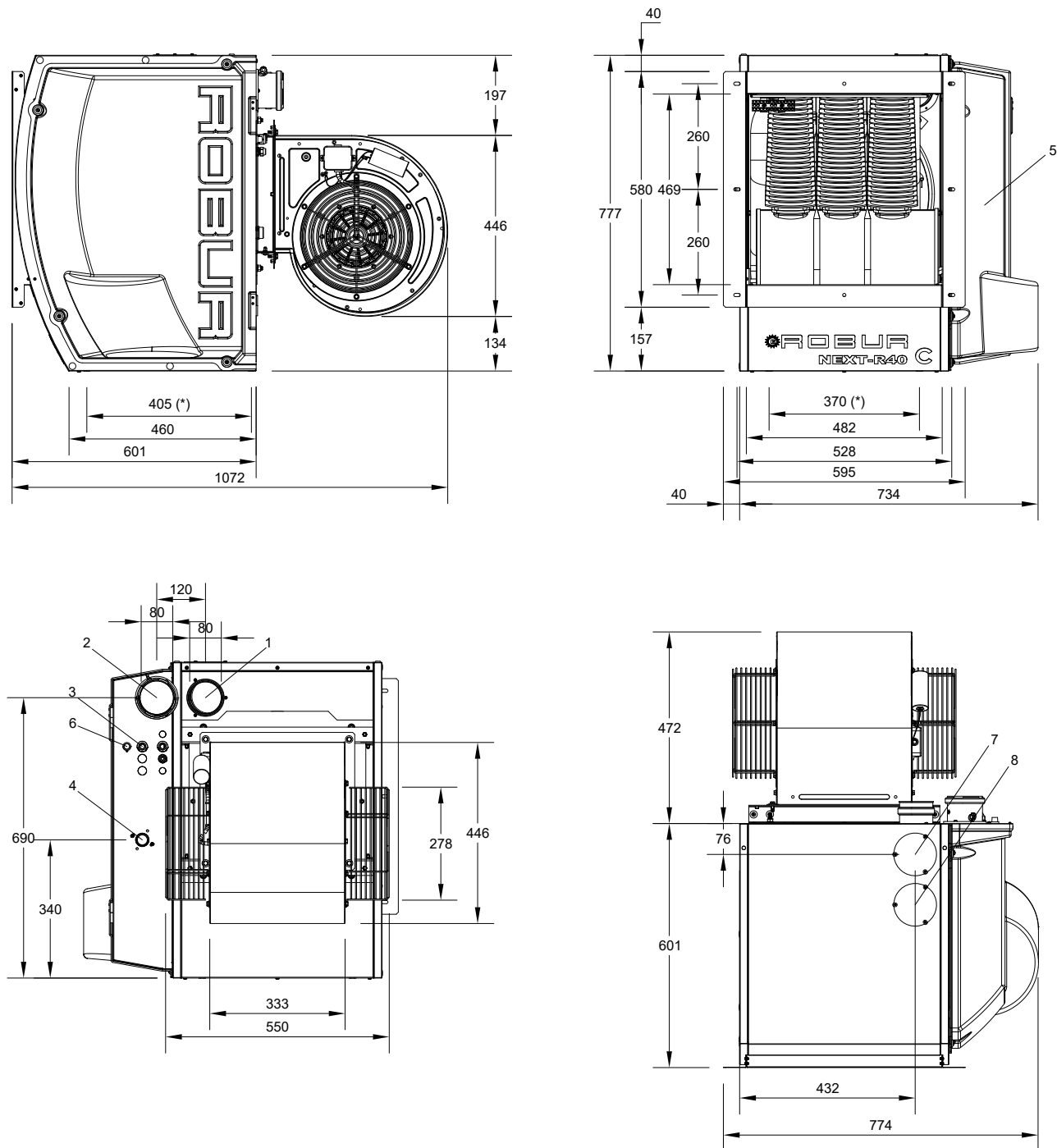
Figura 1.8 Dimensioni unità
