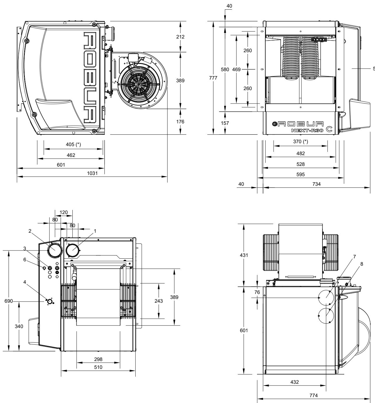
Figura 1.7 Dimensioni unità
