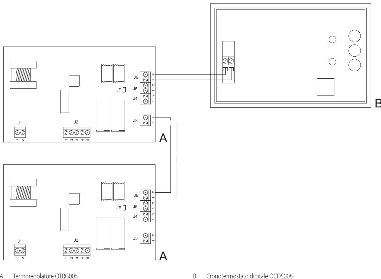
Figura 4.5 Collegamento cronotermostato digitale OCDS008
