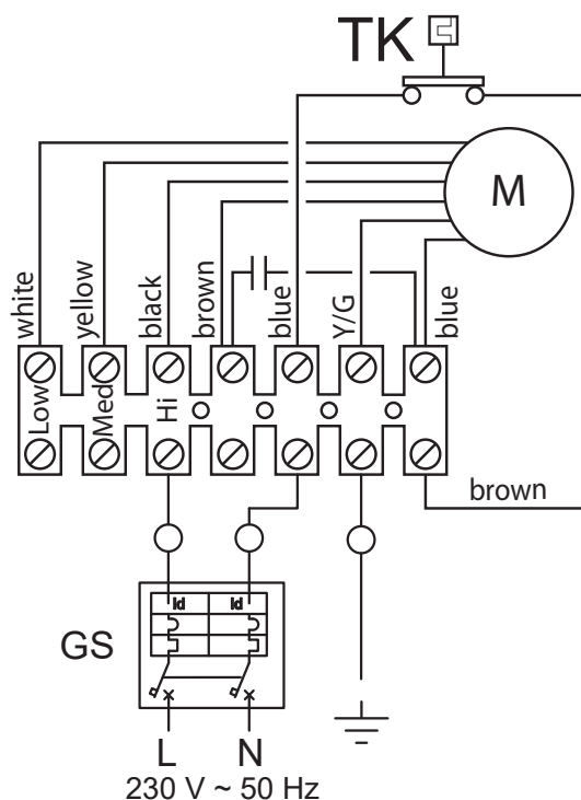
Figura 4.1 Alimentazione elettrica
