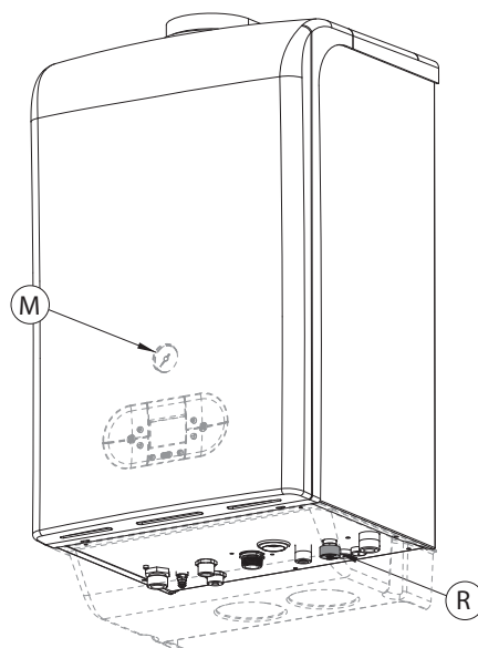
M Manometro R Rubinetto caricamento impianto
