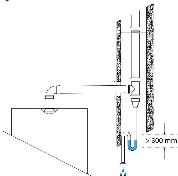
Figura 3.17 Scarico condensa fumi
