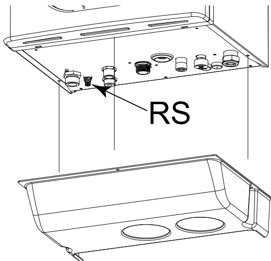
Figura 8.1 Posizione rubinetto di scarico impianto
