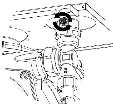
Figura 3.11 Tappo valvola jolly blocco a condensazione
