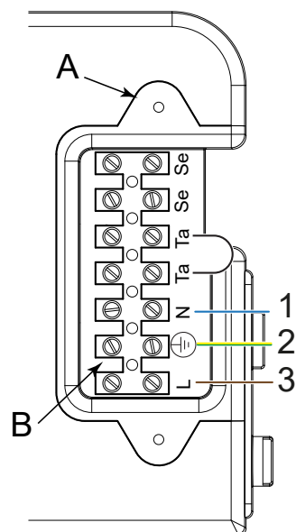
Figura 4.2 Alimentazione elettrica caldaia 35
