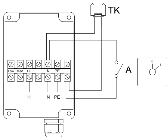
Figura 4.6 Schema collegamenti funzionamento in condizionamento
