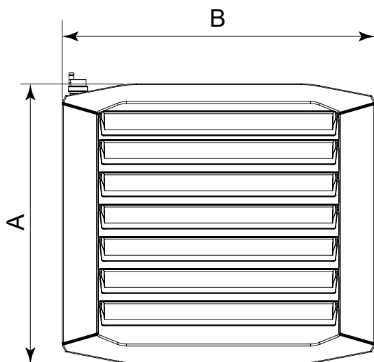
Figura 1.3 Dimensioni aerotermo
