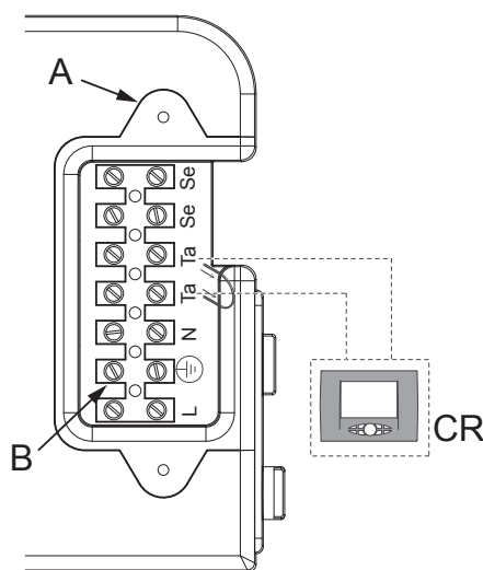
Figura 4.5 Collegamento consenso esterno/termostato ambiente/comando remoto OCDS006 a Caldaia 35
