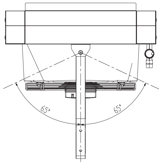
Figura 3.5 Orientamento aerotermo
