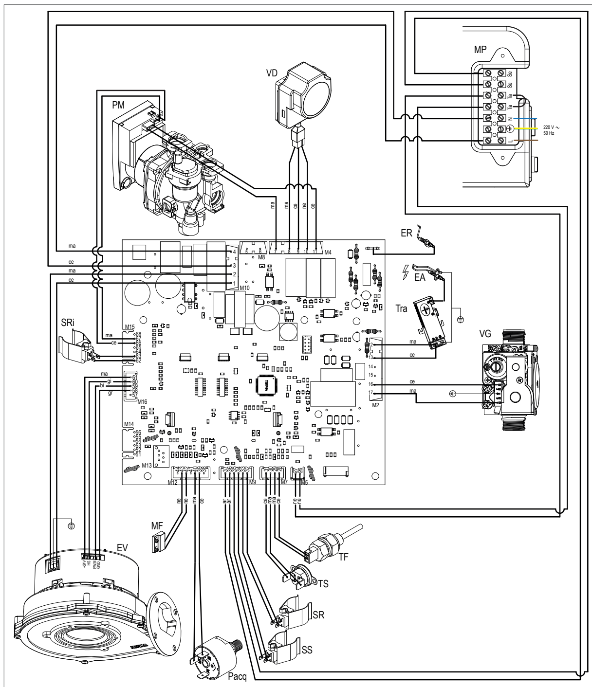
Figura 1.8 Schema collegamenti elettrici caldaia
