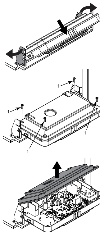
Figura 6.2 Accesso al pannello comandi
