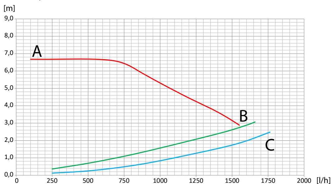
Figura 1.7 Prevalenza e perdite di carico Caldaia 35
