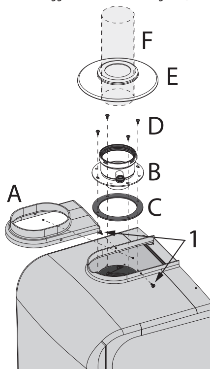
Figura 3.13 Montaggio del tronchetto flangiato (Ø 60/80 mm)
