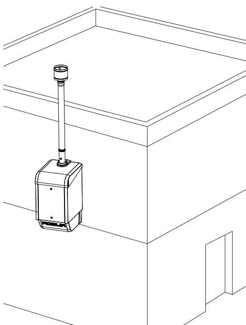
Figura 3.15 Scarico fumi verticale a tetto
