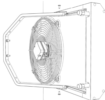
Figura 3.4 Fissaggio staffa all'aerotermo
