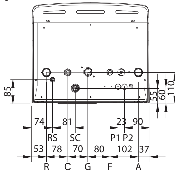
Figura 1.2 Attacchi idraulici Caldaria 35 ACS (vista inferiore)
