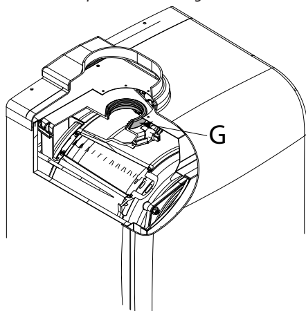
Figura 3.14 Corretto posizionamento guarnizione
