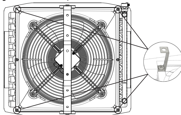
Figura 3.2 Staffe di sospensione verticale
