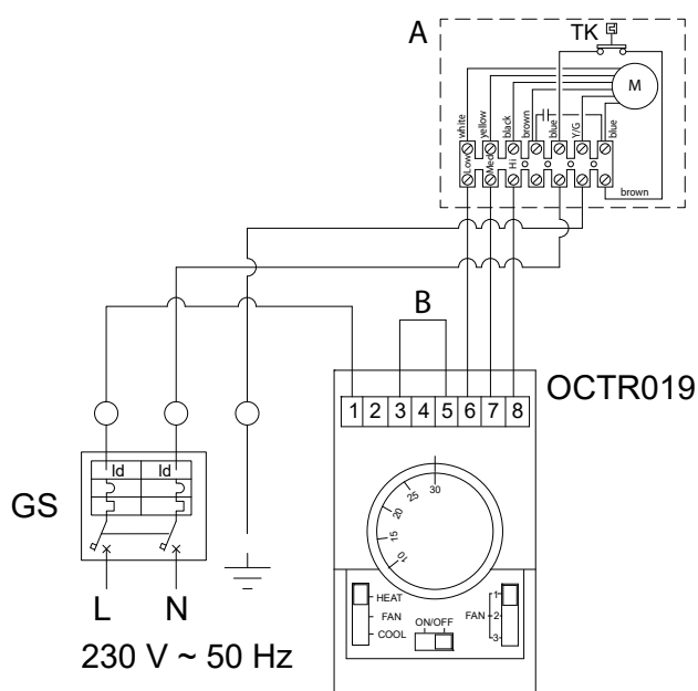
Figura 4.3 Aerotermo Tech con comando a terra OCTR019, con termostato ambiente attivo
