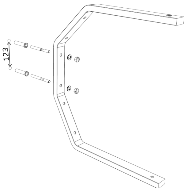
Figura 3.3 Posizione fori aerotermo
