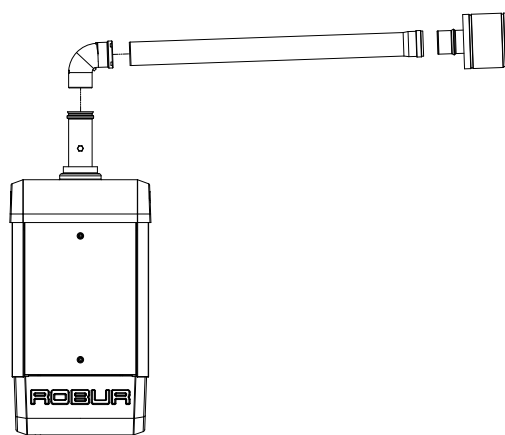
Figura 3.16 Scarico fumi orizzontale
