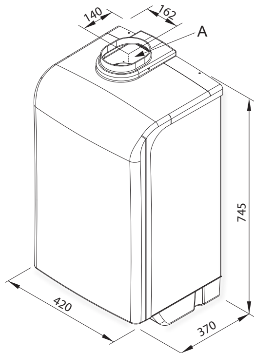
Figura 1.1 Dimensioni Caldaria 35
