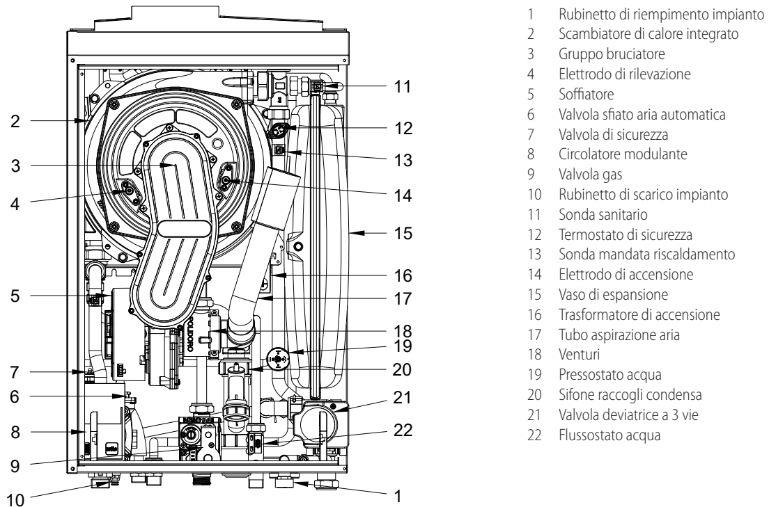
Figura 1.4 Vista frontale interna caldaia
