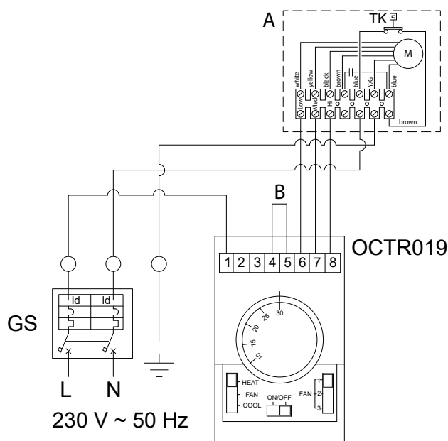
Figura 4.4 Aerotermo Tech con comando a terra OCTR019, con termostato ambiente disattivato
