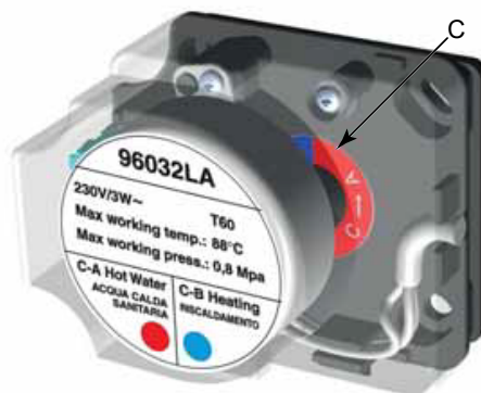
Figura 8.2 Valvola deviatrice
