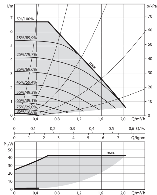
Figura 1.6 Curve caratteristiche circolatore
