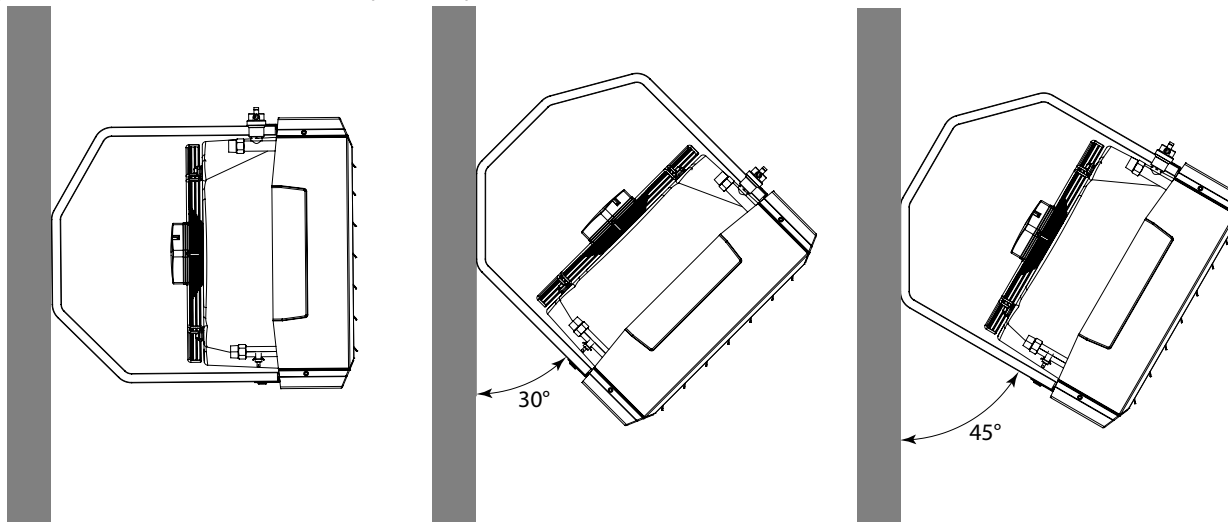
Figura 3.6 Posizionamento aerotermo rispetto alla parete
