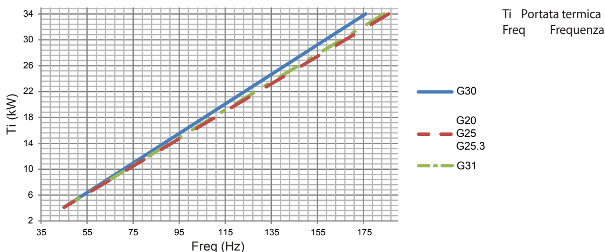
Figura 6.4 Diagramma portata termica/frequenza soffiatore
