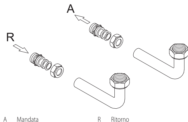
Figura 3.8 Kit raccordi idronici
