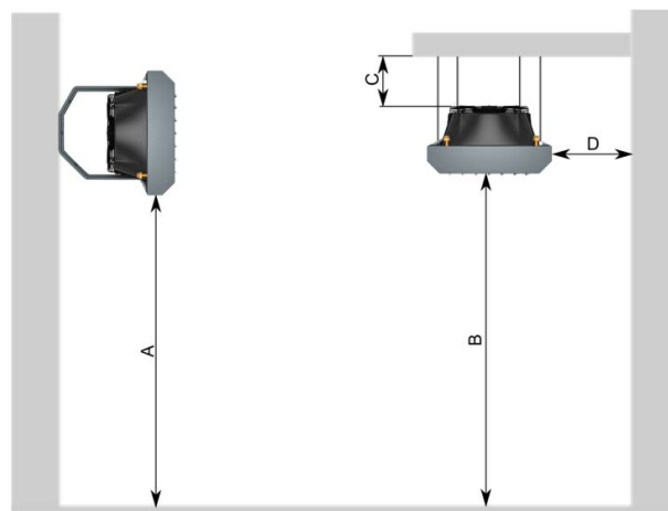
Figura 2.2 Distanze minime di rispetto
