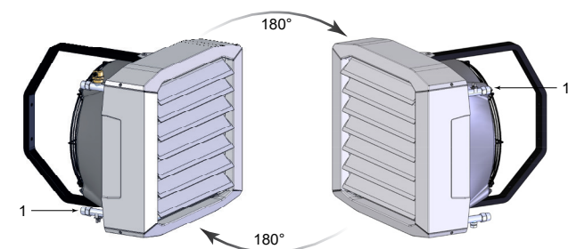
Figura 3.1 Rotazione aerotermo
