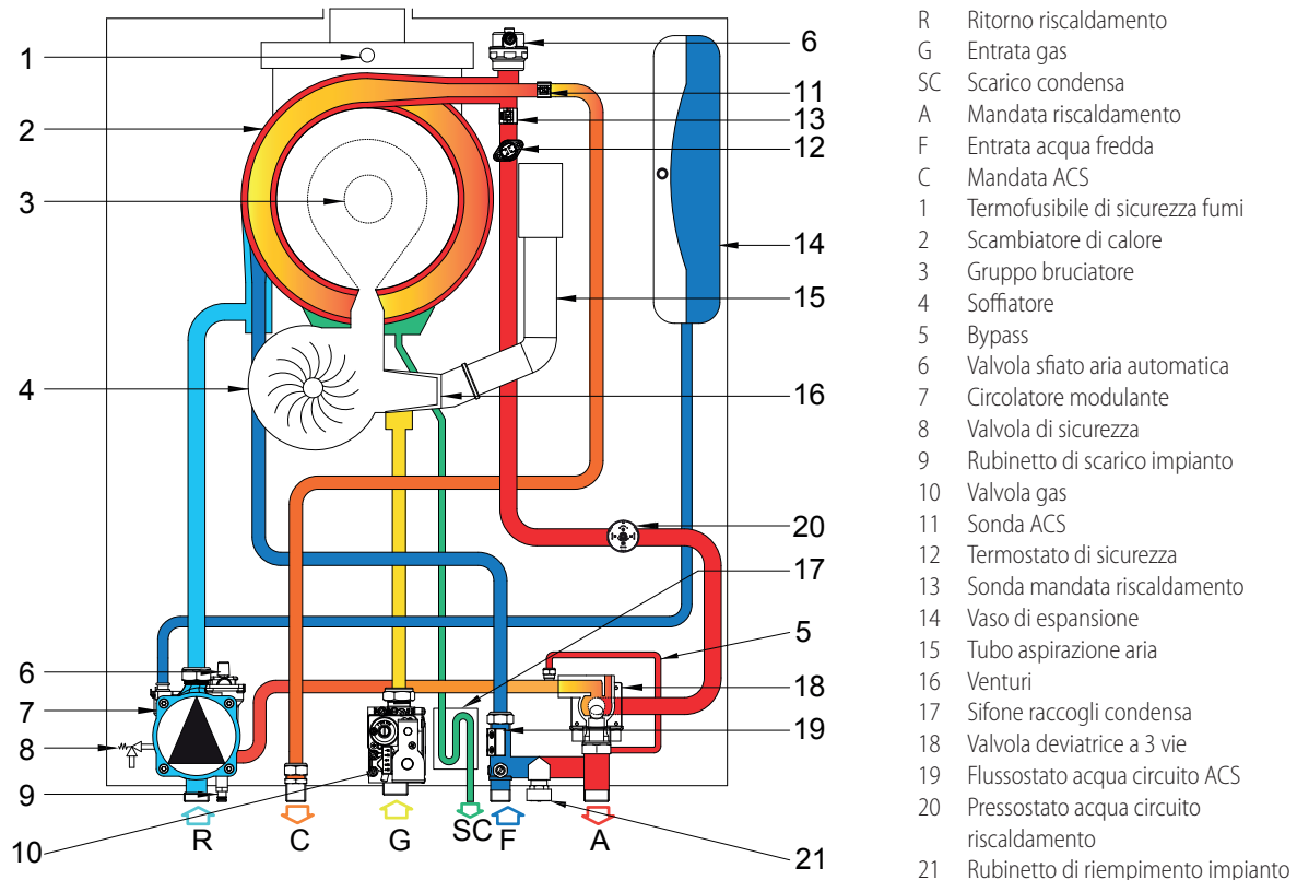
Figura 1.5 Schema idraulico interno caldaia
