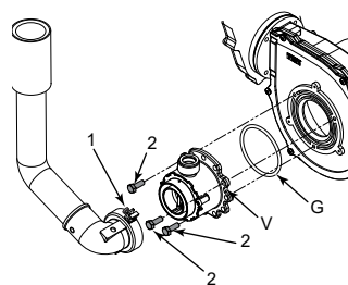
Figura 6.7 Cambio gas
