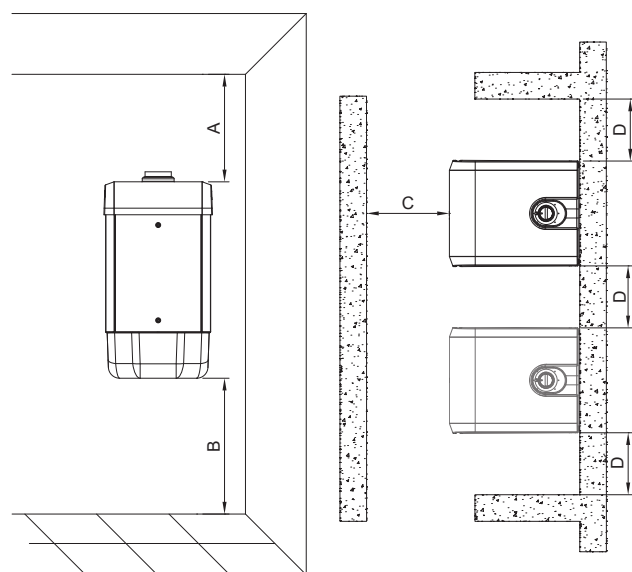
Figura 2.1 Distanze minime di rispetto
