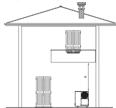
Figura 2.4 Zona aperta minima sopra le unità
