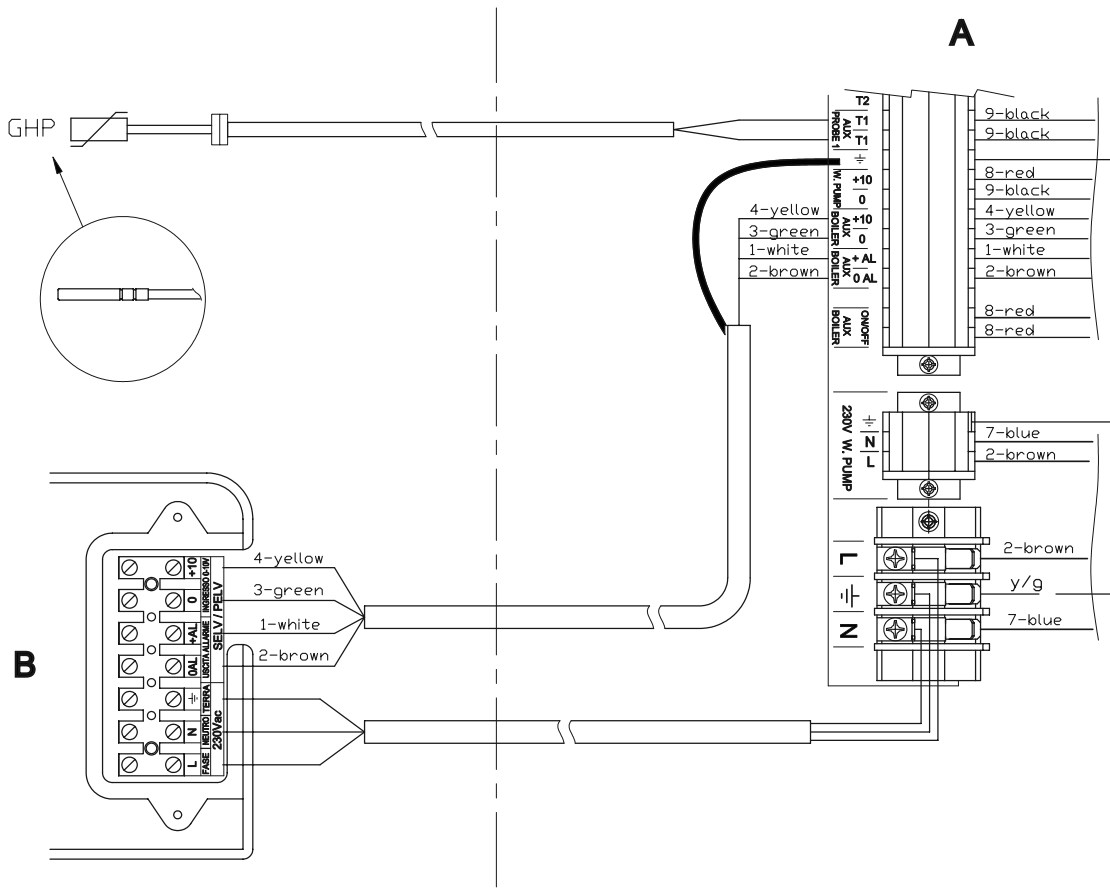
Figura 1.14 Dettaglio collegamento tra quadro elettrico modulo pompa di calore e quadro elettrico modulo caldaia
