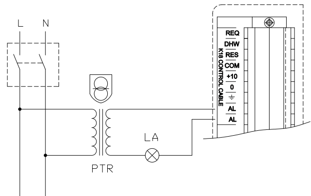
Figura 4.6 Collegamento lampada di segnalazione allarmi
