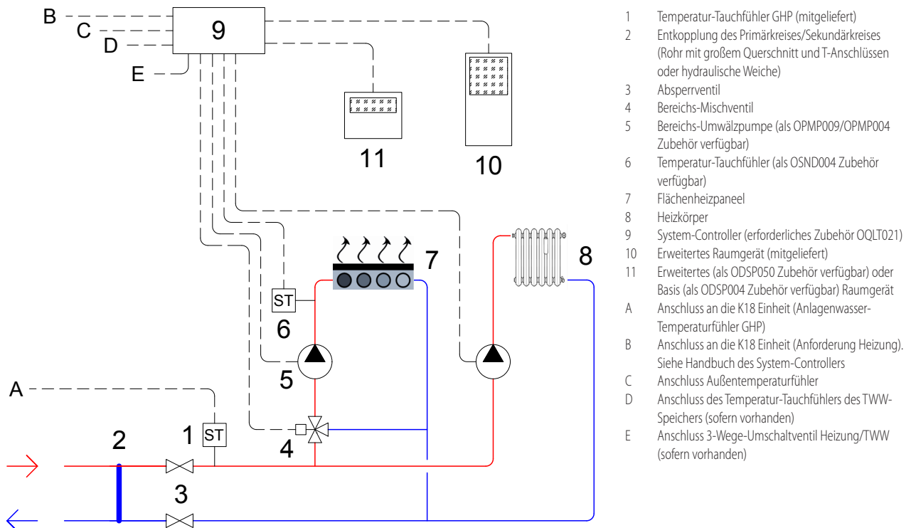
Abbildung 3.6 Heizungsverteiler 03 - System-Controller mit einem gemischten und einem direkten Heizkreis
