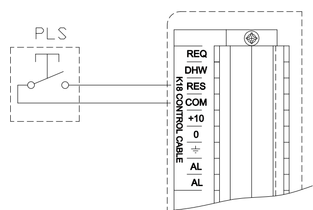
Abbildung 4.10 Anschluss der Fehler-Resets der Steuerplatine
