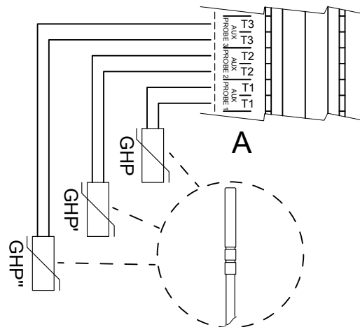
Abbildung 4.12 Anschluss von Temperaturfühlern ans K18-Gerät, mit direkt vom Gerät gesteuertem TWW, mit einem Hilfswärmeerzeuger
