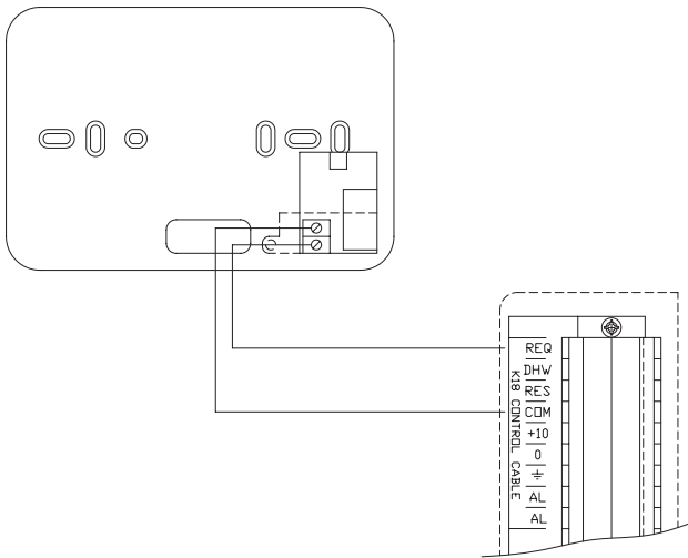
Abbildung 4.3 Anschluss der Betriebsfreigabe an den Thermostat mit Zeitschaltuhr OCDS007
