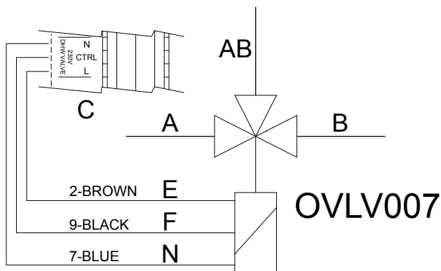
Abbildung 4.7 Anschluss des TWW-Umschaltventils OVLV007
