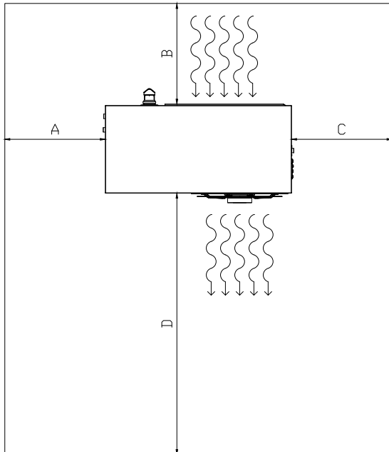
Abbildung 2.3 K18 Simplygas Mindestabstände
