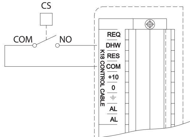
Abbildung 4.6 Anschluss der externen Freigabe für das TWW
