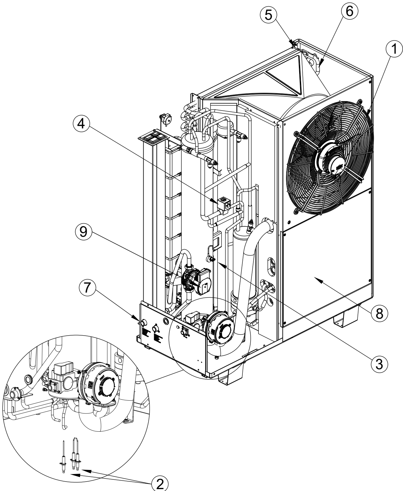
Abbildung 1.4 Interne Komponenten des Wärmepumpenmoduls Vorderansicht links
