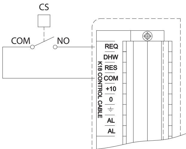
Abbildung 4.5 Anschluss der externen Freigabe für die Heizung
