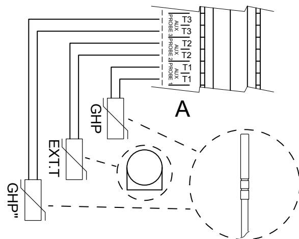
Abbildung 4.13 Anschluss von Temperaturfühlern ans K18-Gerät, mit direkt vom Gerät gesteuertem TWW, ohne Hilfswärmeerzeuger
