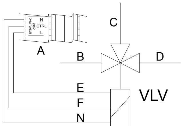
Abbildung 4.8 Anschluss eines allgemeinen TWW-Umschaltventils
