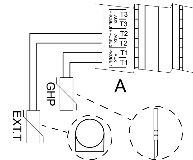
Abbildung 4.11 Anschluss von Temperaturfühlern ans K18-Gerät nur für den Heizbetrieb
