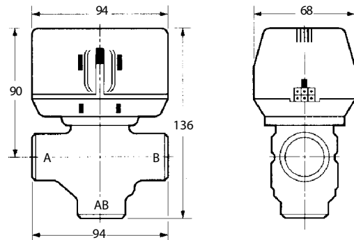
Abbildung 3.7 Abmessungen Umschaltventil OVLV007
