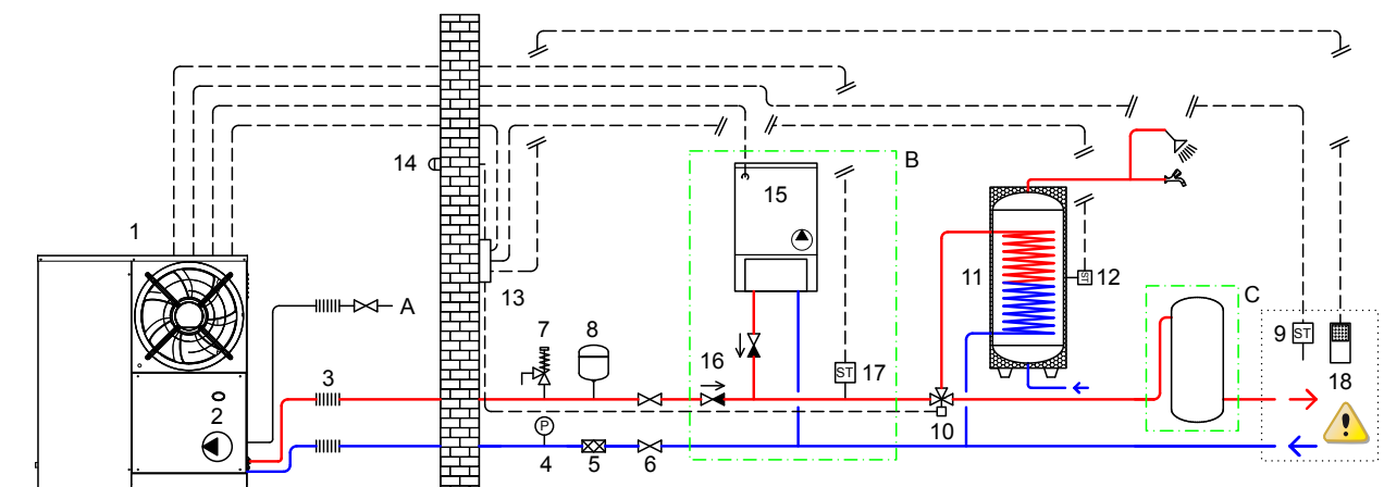
Abbildung 3.3 K18 Simplygas C1 mit OQLT021 System-Controller, mit optionalem Hilfswärmeerzeuger
