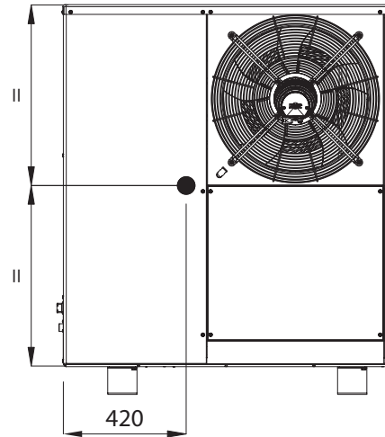
Abbildung 2.2 Schwerpunktposition Einheit
