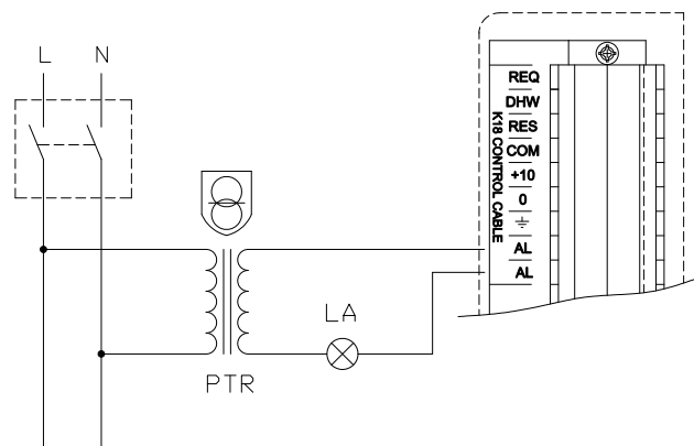
Abbildung 4.9 Anschluss der optischen Alarmanzeige
