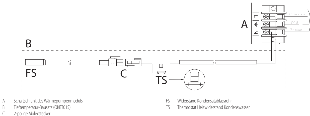
Abbildung 4.15 Anschluss des Tieftemperatur-Bausatzes für K18 Simplygas
