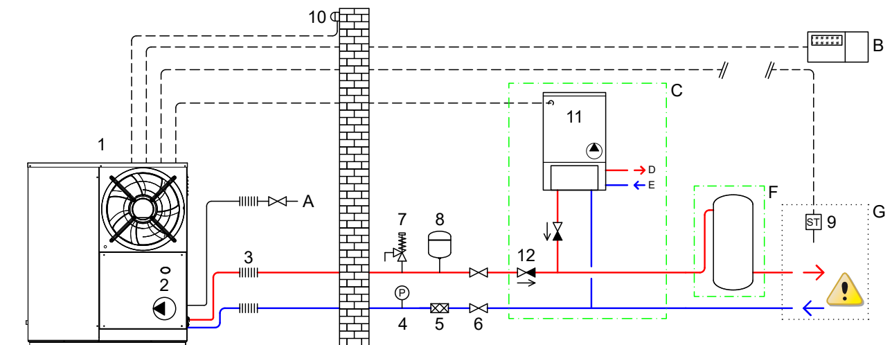
Abbildung 3.1 K18 Simplygas C1 nur für Heizung, mit optionalem Hilfswärmeerzeuger
