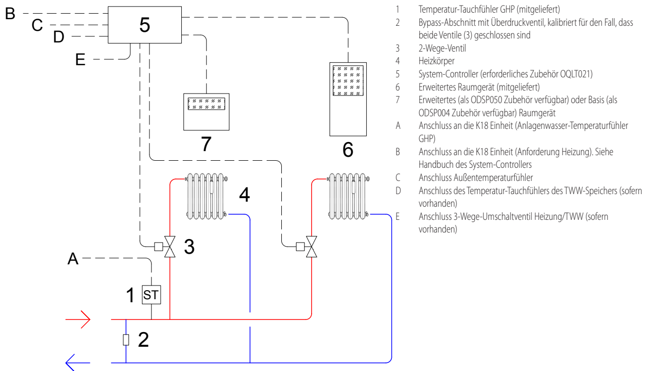
Abbildung 3.5 Heizungsverteiler 02 - System-Controller mit zwei 2-Wege-Bereichsventilen
