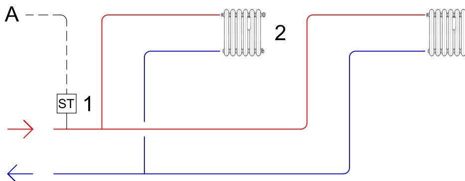
Abbildung 3.4 Heizungsverteiler 01 - direkt
