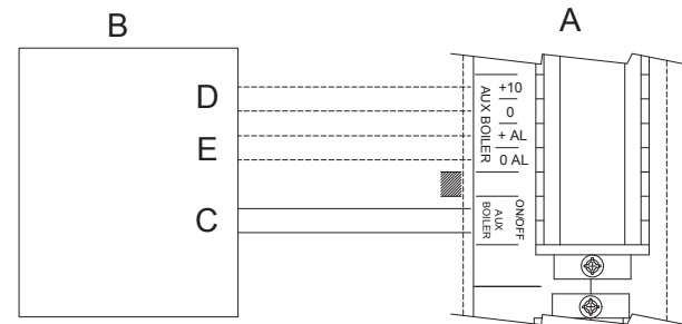
Abbildung 4.14 Anschluss Freigabe Ein/Aus und eventueller Ausgang 0-10 V (Sollwert Temperatur) und mögliches Alarmsignal für Hilfswärmeerzeuger am Klemmbrett der Einheit
