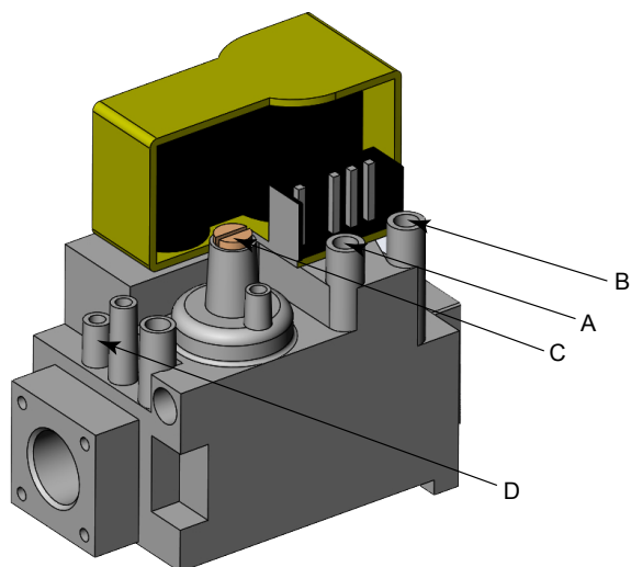
Abbildung 5.1 Gasventil Wärmepumpenmodul
