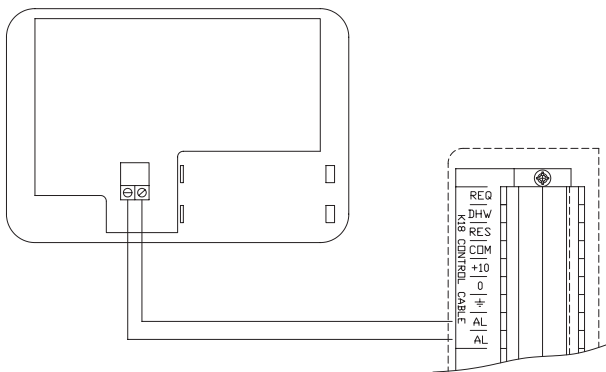
Abbildung 4.4 Anschluss des Alarmanzeigesignals an den Thermostat mit Zeitschaltuhr OCDS007
