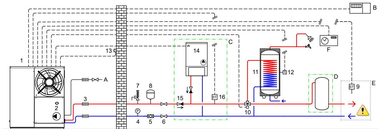
Abbildung 3.2 K18 Simplygas C1 für Heizung und TWW-Erzeugung (Basisfunktionalität), mit optionalem Hilfswärmeerzeuger
