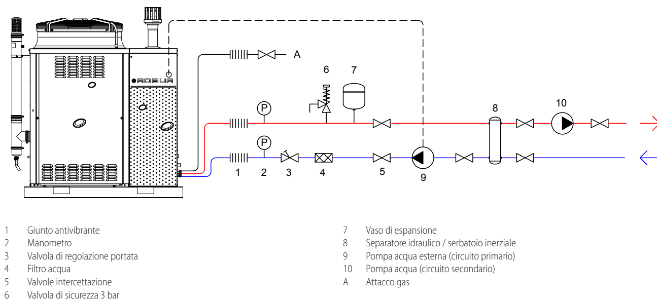
Figura 3.1 Schema idraulico Gitié ARAY /2 C0
