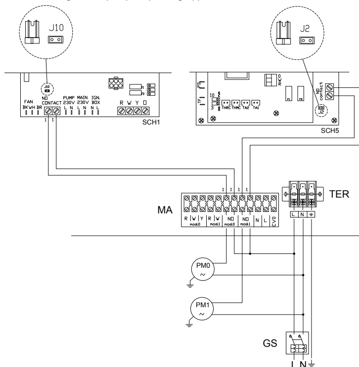
Figura 4.7 Schema collegamento pompe impianto gruppo Gitié versione base ( P < 700\text{ W} )
