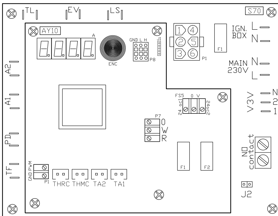
Figura 1.17 Schede elettroniche AY10+S70
