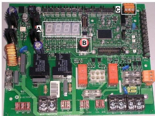
Figura 5.1 Scheda elettronica S61 a bordo unità GAHP/GA
