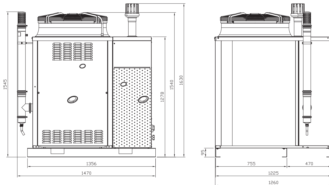
Figura 1.2 Dimensioni (ventilatore silenzioso)
