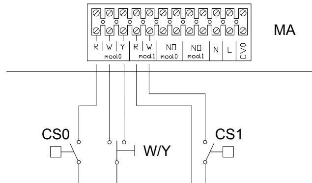
Figura 4.6 Schema collegamento consensi esterni caldo separati
