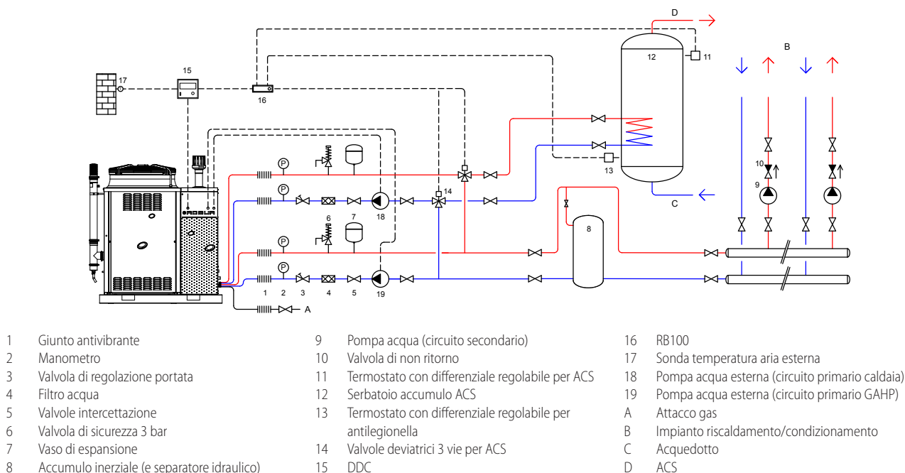
Figura 3.2 Schema idraulico Gitié ARAY /4 C0 ACS
