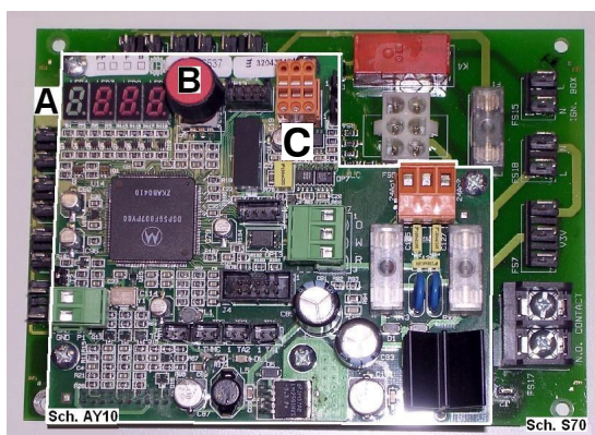
Figura 5.2 Scheda elettronica (AY10+S70) a bordo unità AY00-120
