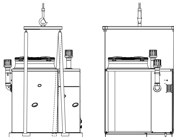
Figura 2.1 Indicazioni per il sollevamento
