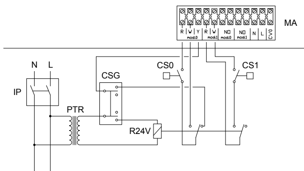
Figura 4.5 Schema collegamento consensi esterni caldo contemporanei
