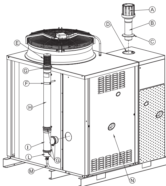
Figura 3.3 Scarico fumi
