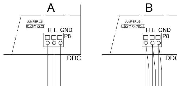
Figura 4.4 Connessione cavo CAN bus al pannello di controllo
