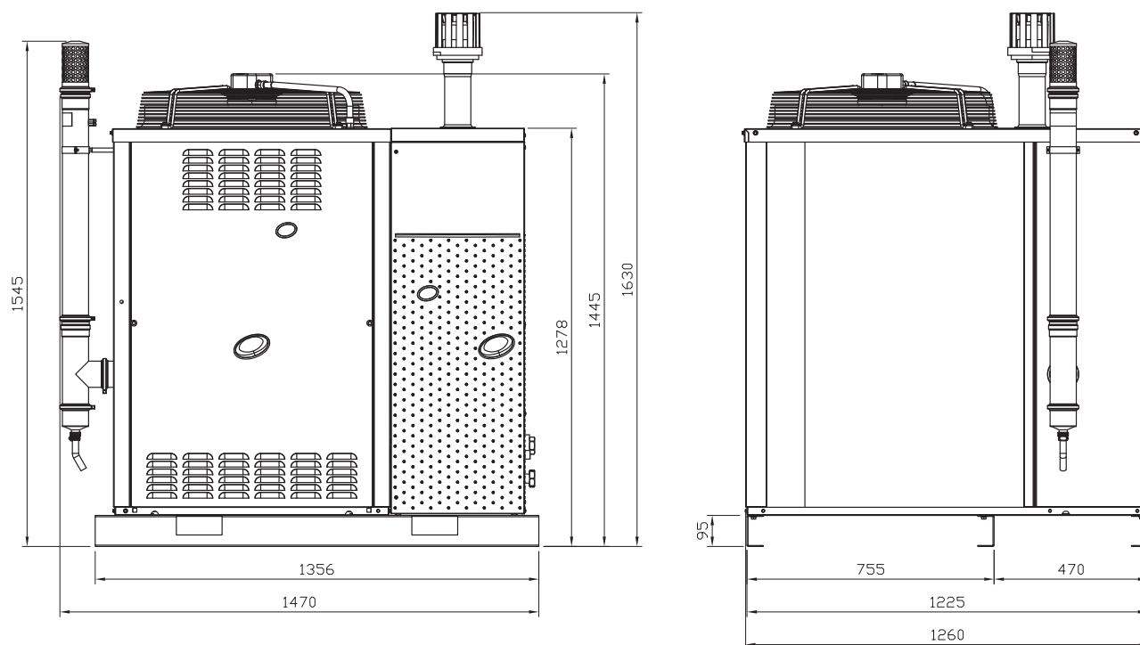
Figura 1.1 Dimensioni (ventilatore standard)
