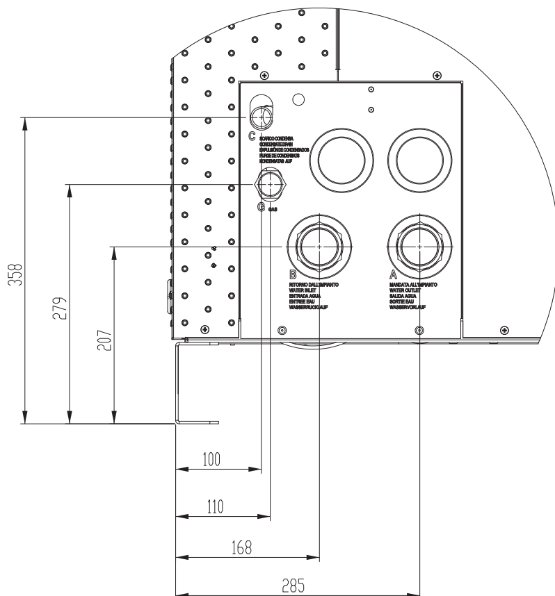
Figura 1.3 Piastra servizi gruppo 2 tubi (KIT/2 C0 e C1) - Dettaglio attacchi idraulici/gas
