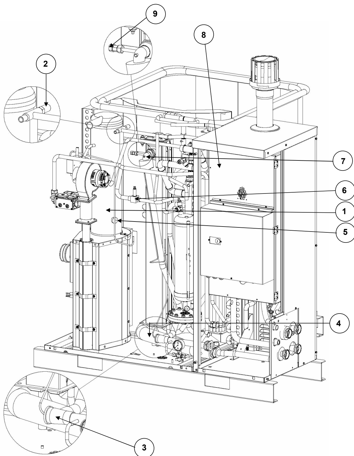
Figura 1.8 Componenti interni vista lato destro
