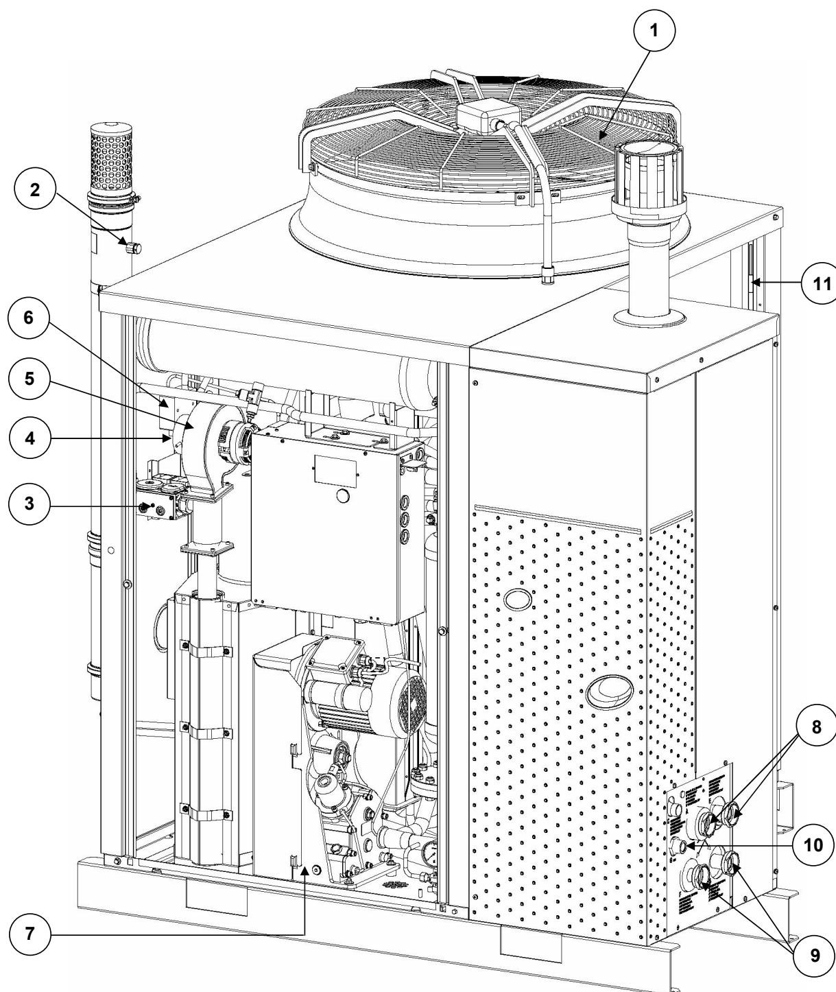
Figura 1.5 Componenti interni vista frontale
