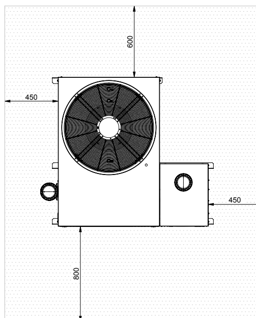
Figura 2.2 Distanze di rispetto
