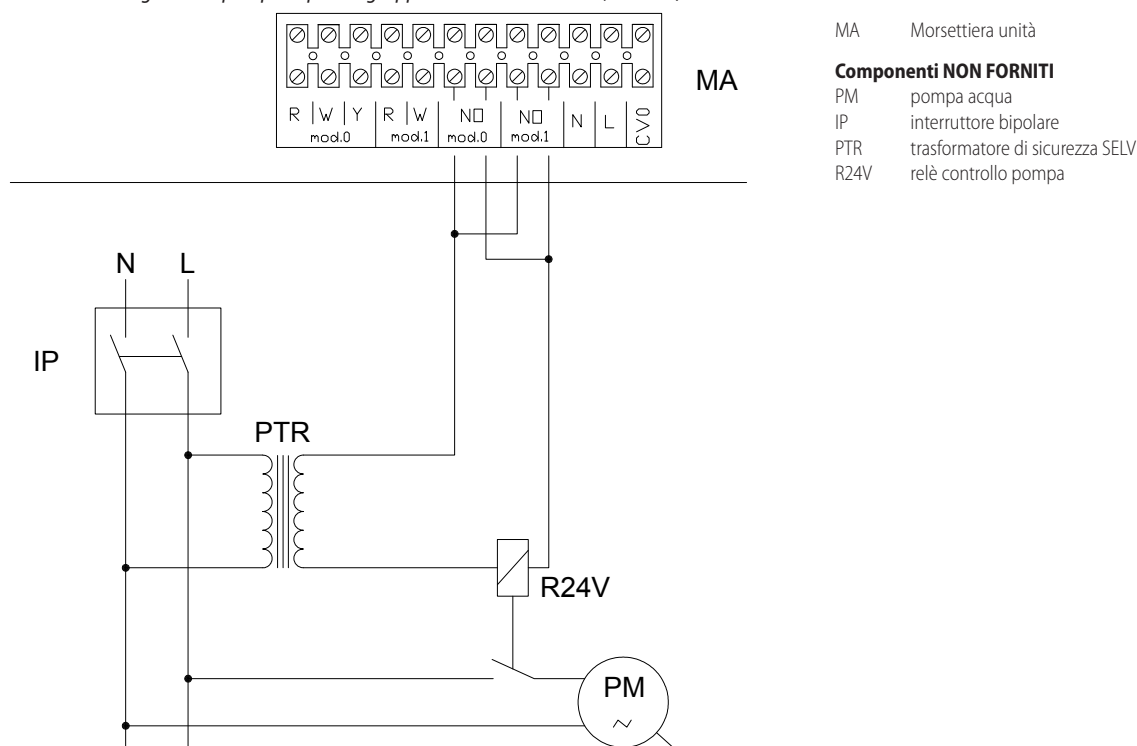
Figura 4.8 Schema collegamento pompe impianto gruppo Gitié versione 2 tubi (KIT/2 C0)
