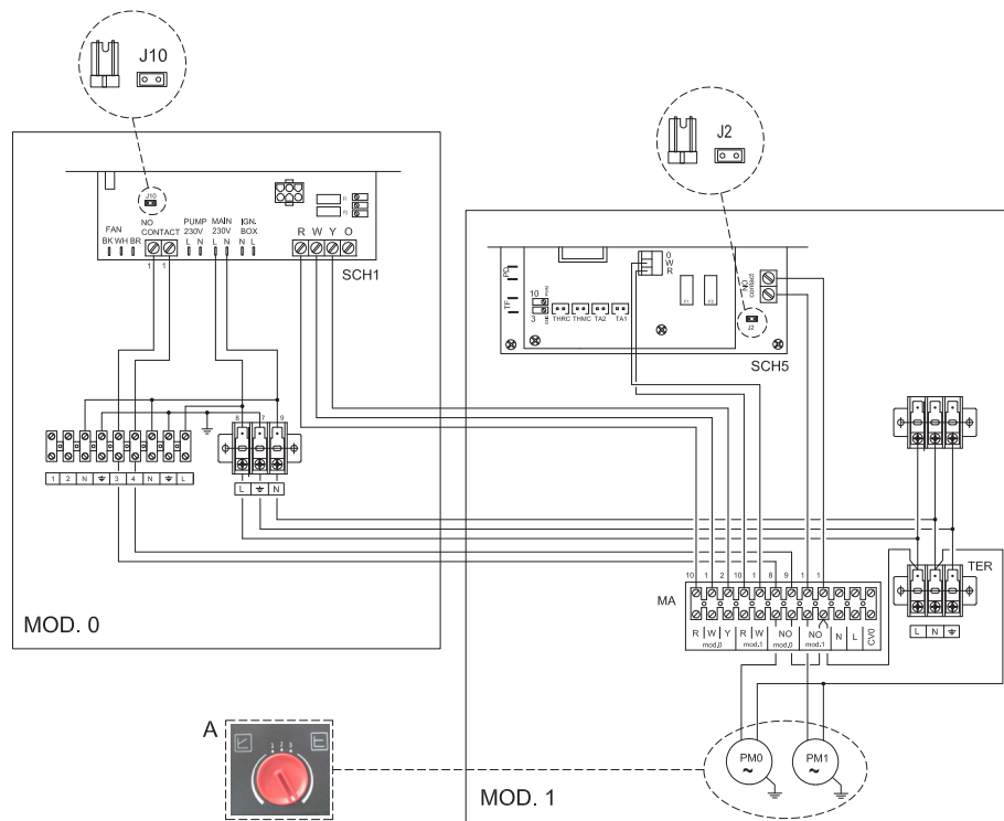
Figura 1.13 Schema elettrico dei gruppi Gitié con KIT/2 C1 o con KIT/4 C1
