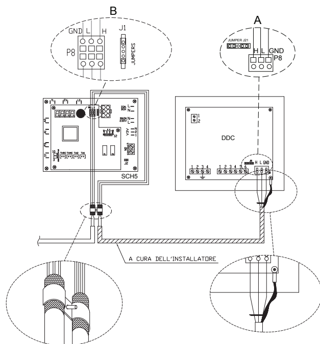
Figura 4.3 Collegamento CAN-BUS tra Gitié e DDC
