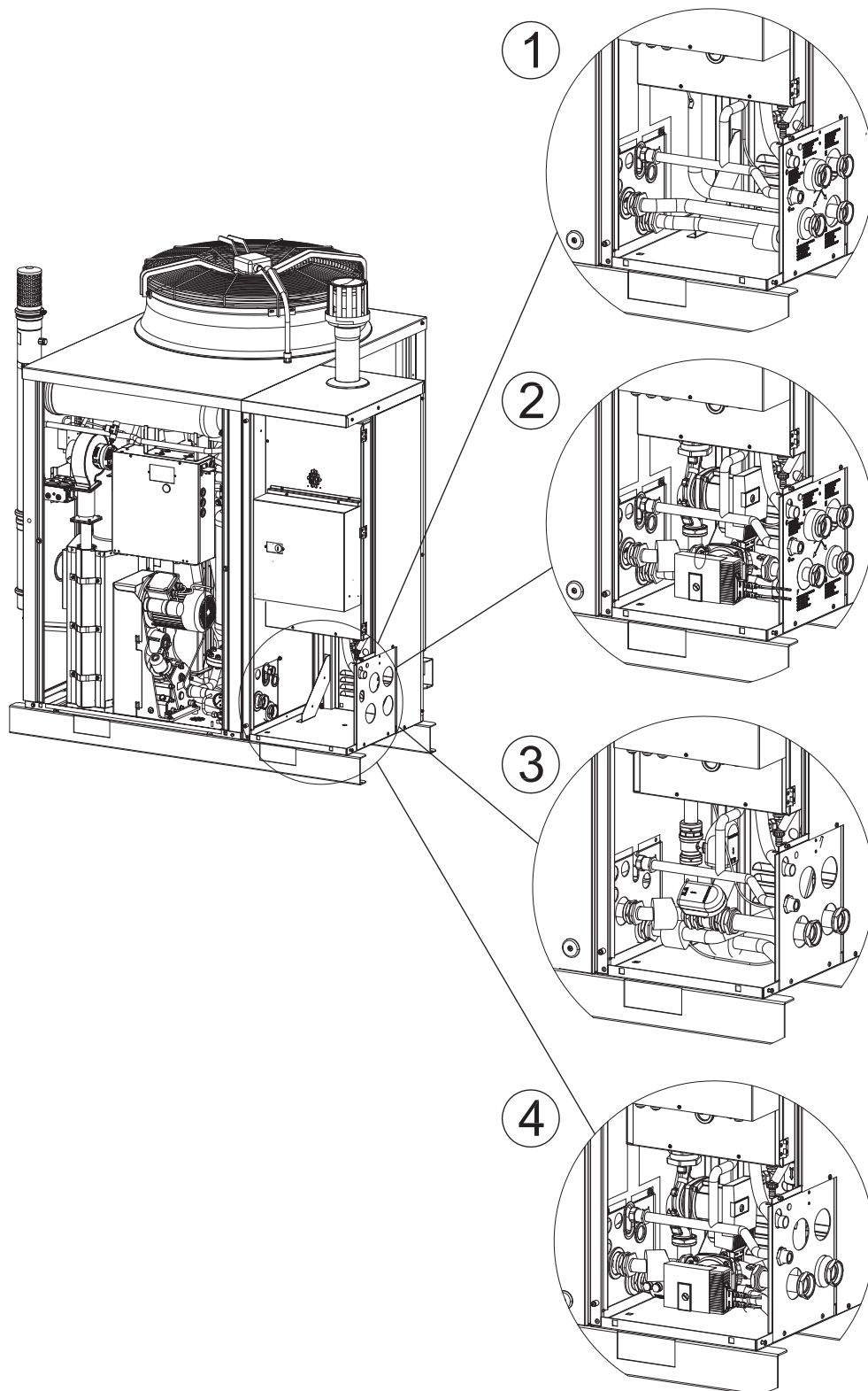
Figura 1.6 Componenti versioni
