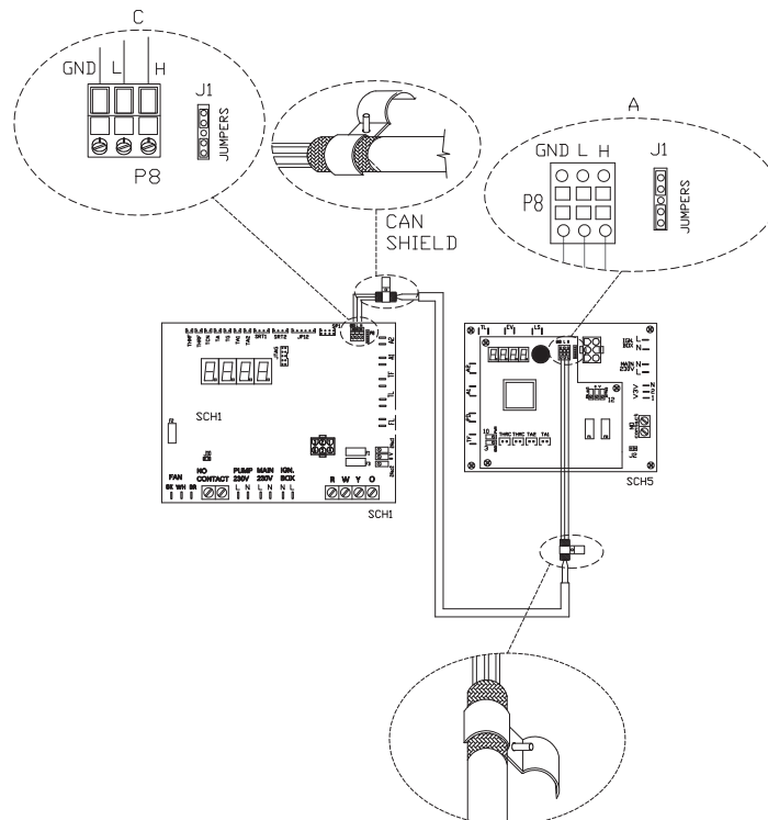
Figura 1.14 Collegamento CAN tra scheda AY10 e S61 (precablato in fabbrica)
