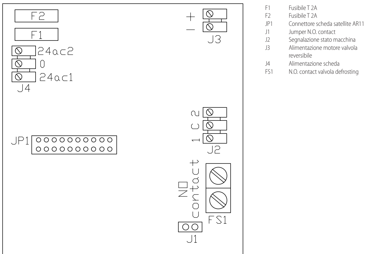
Figura 1.16 Scheda elettronica AR11
