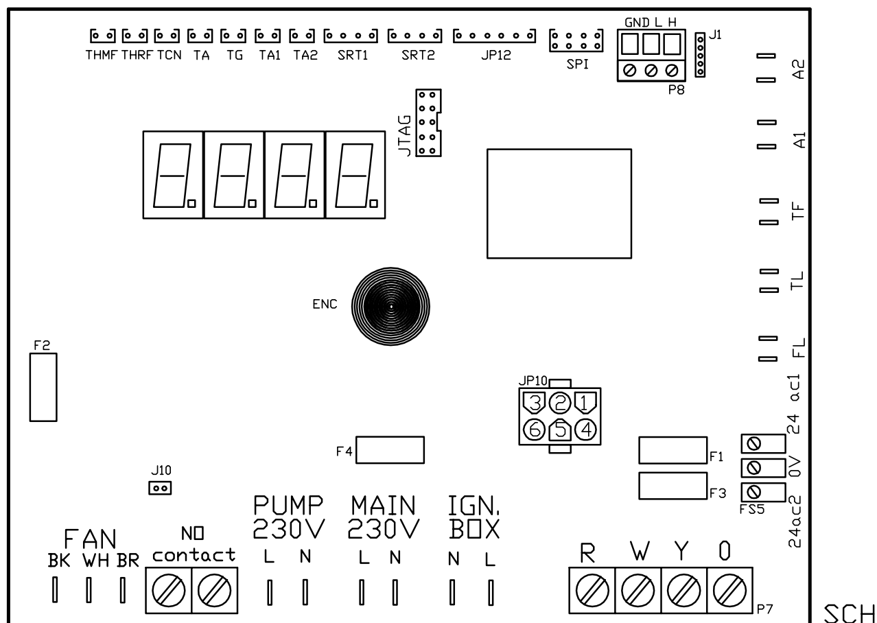
Figura 1.15 Scheda elettronica S61
