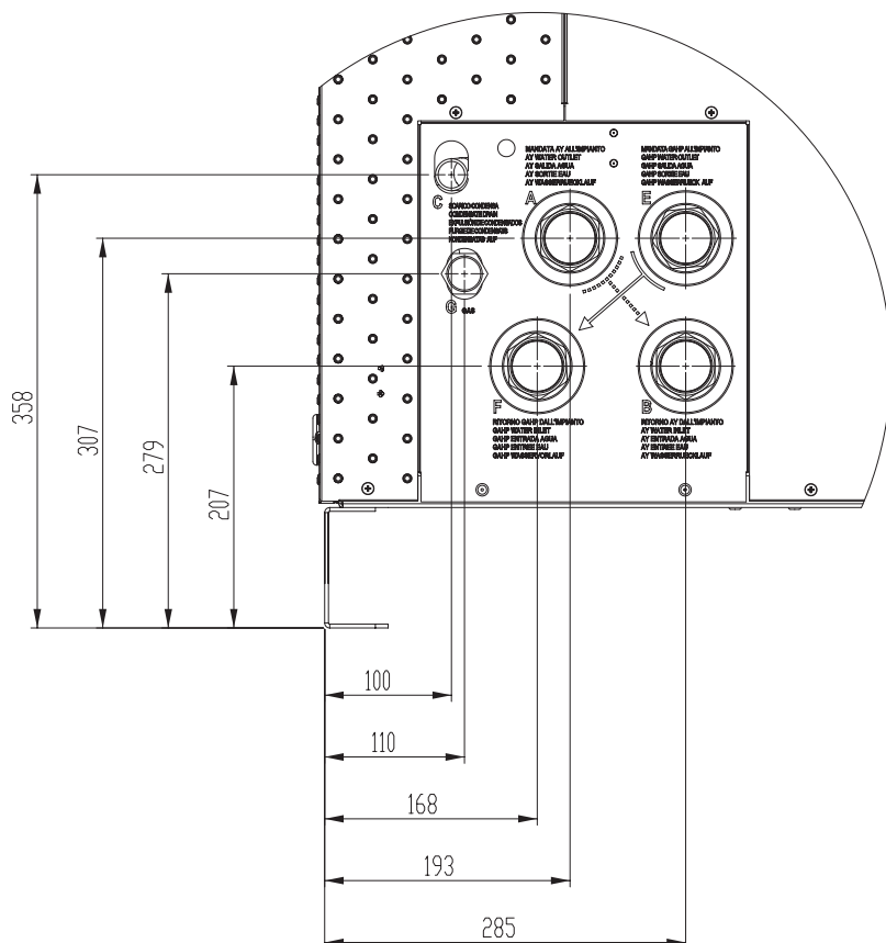
Figura 1.4 Piastra servizi gruppo 4 tubi (versione base e KIT/4 C1) - Dettaglio attacchi idraulici/gas
