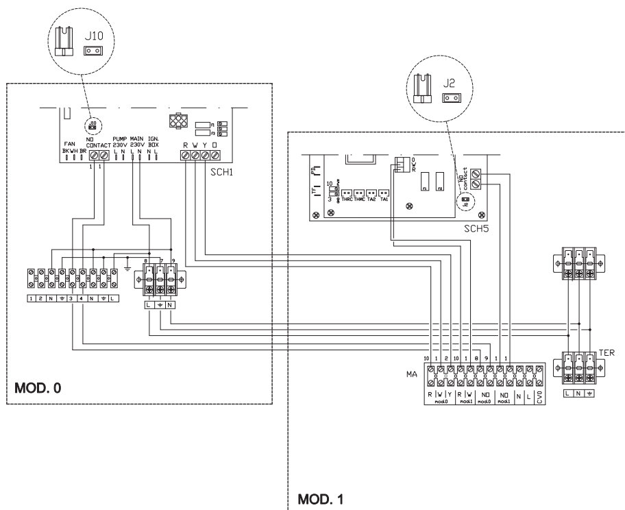
Figura 1.11 Schema elettrico del gruppo Gitié - versione base
