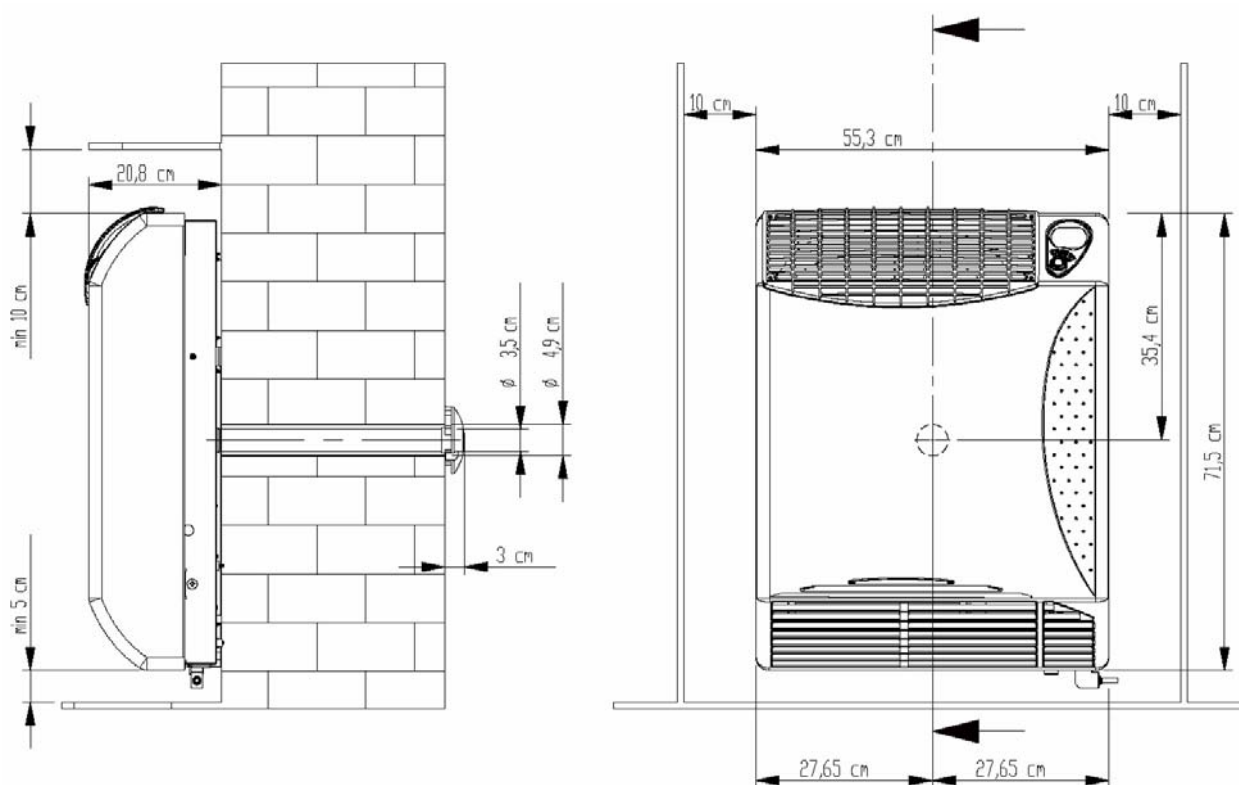
Abbildung 1 – Abmessungen der Heizkörper Calorio
