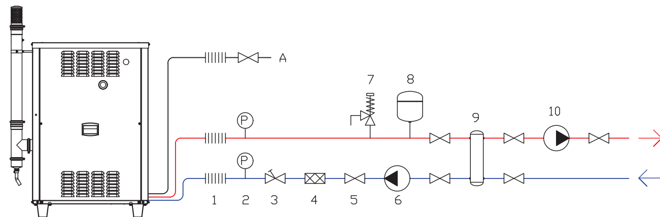
Figura 3.1 Schema idraulico
