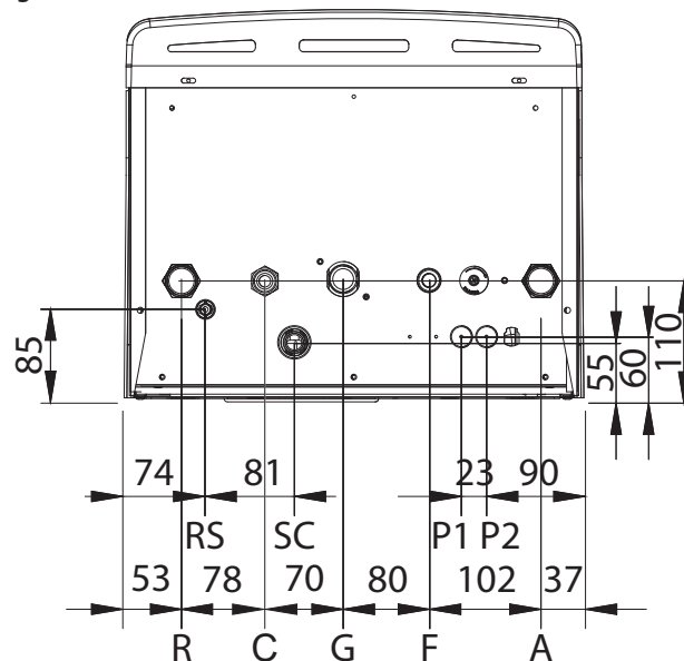
Figura 3.2 Attacchi idraulici Caldaia 35 ACS (vista inferiore)
