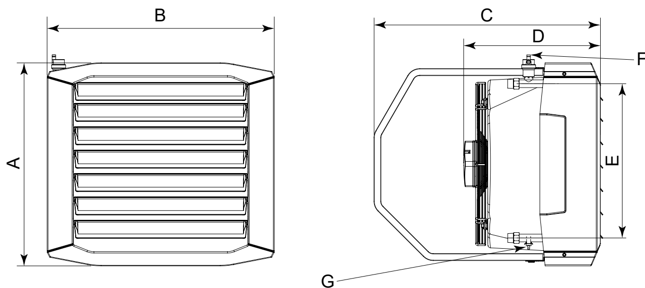
Figura 3.3 Dimensioni aerotermo
