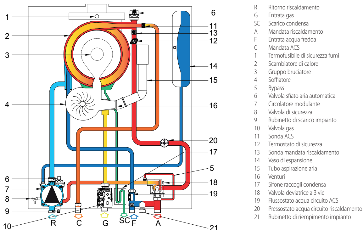
Figura 3.5 Schema idraulico interno caldaia
