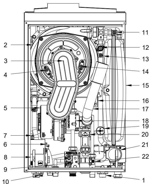
Figura 3.4 Vista frontale interna caldaia
