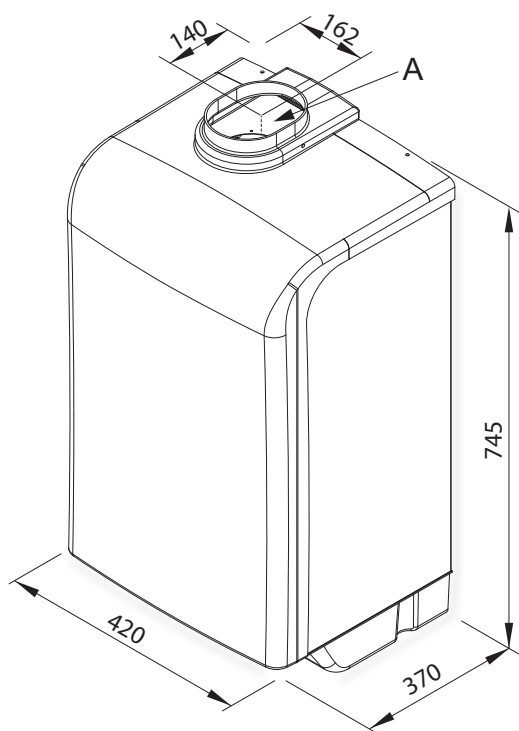
Figura 3.1 Dimensioni Caldaia 35
