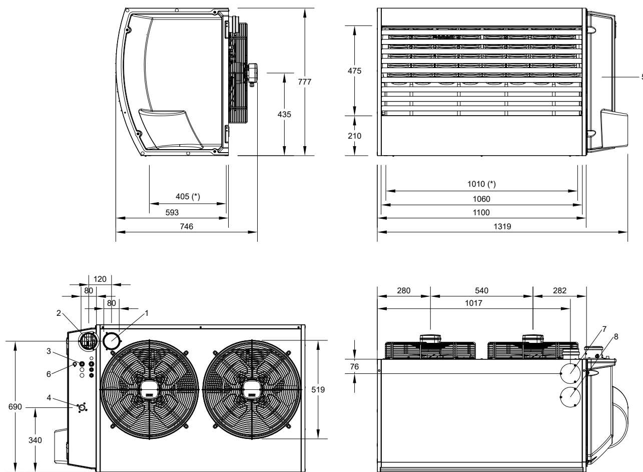
Figura 4.6 Dimensioni unità
