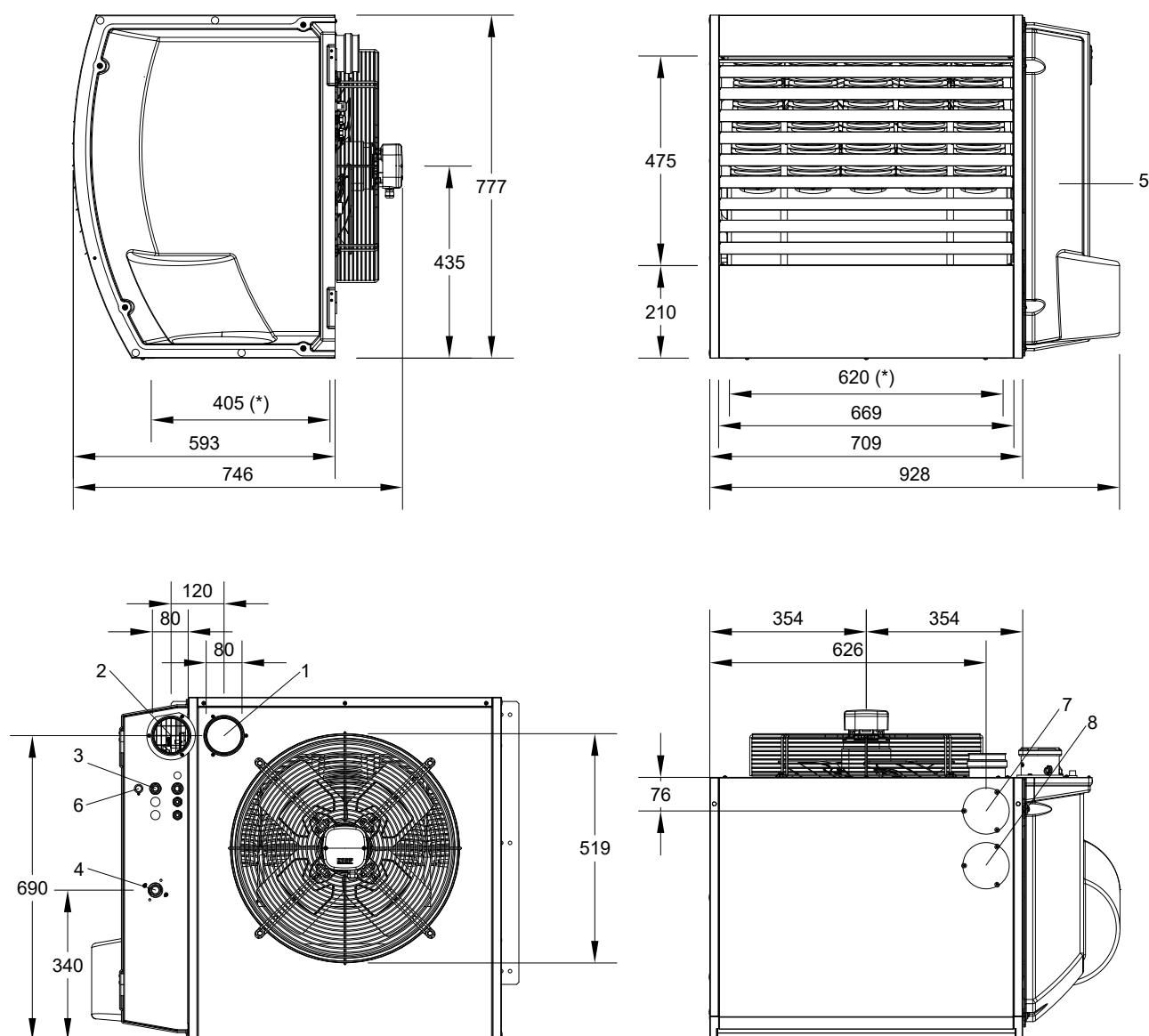
Figura 4.4 Dimensioni unità
