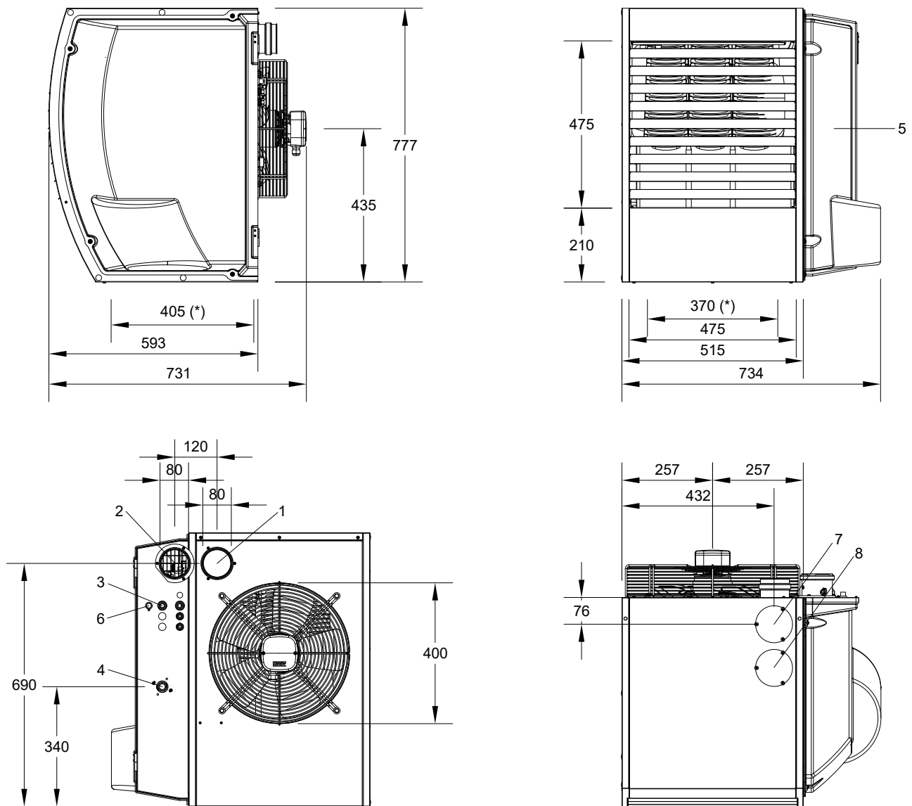
Figura 4.3 Dimensioni unità
