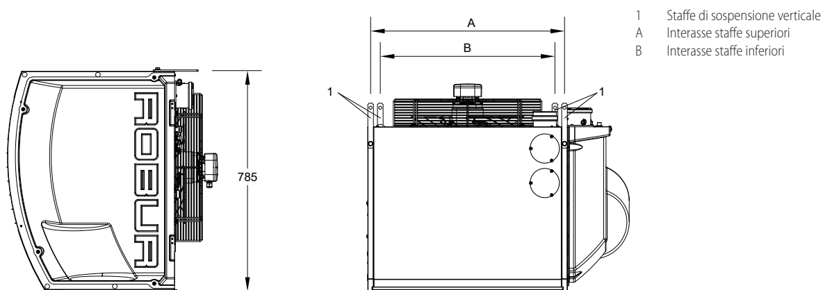
Figura 4.11 Posizione staffe generatori a lancio verticale
