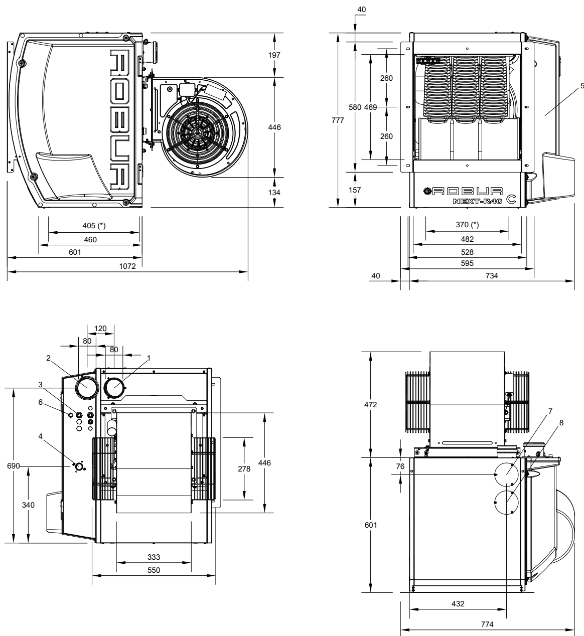
Figura 4.8 Dimensioni unità
