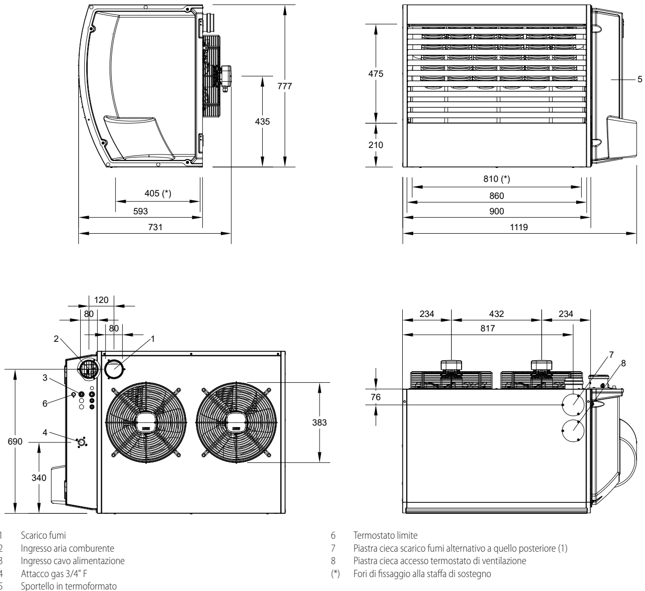
Figura 4.5 Dimensioni unità
