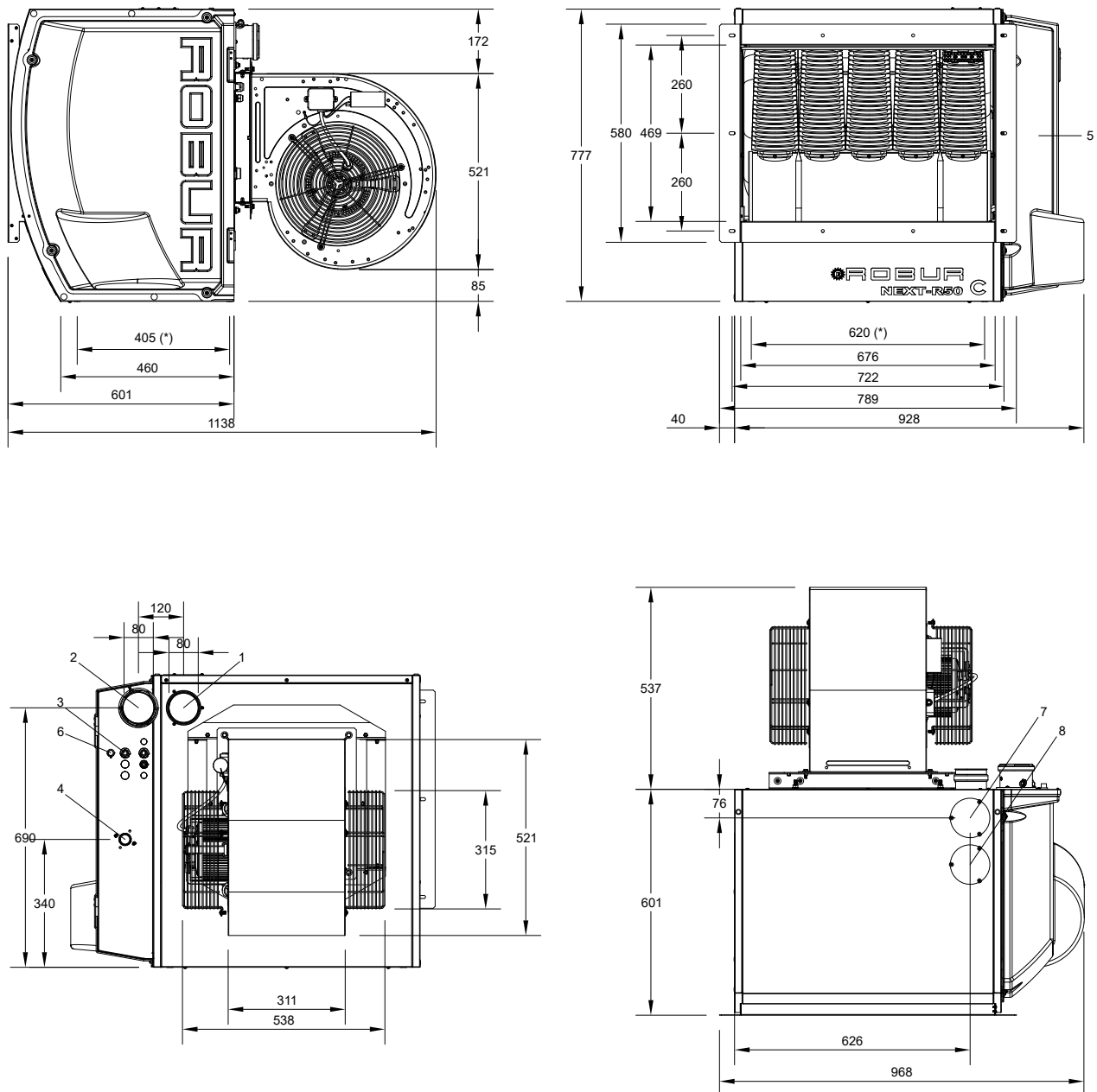
Figura 4.9 Dimensioni unità
