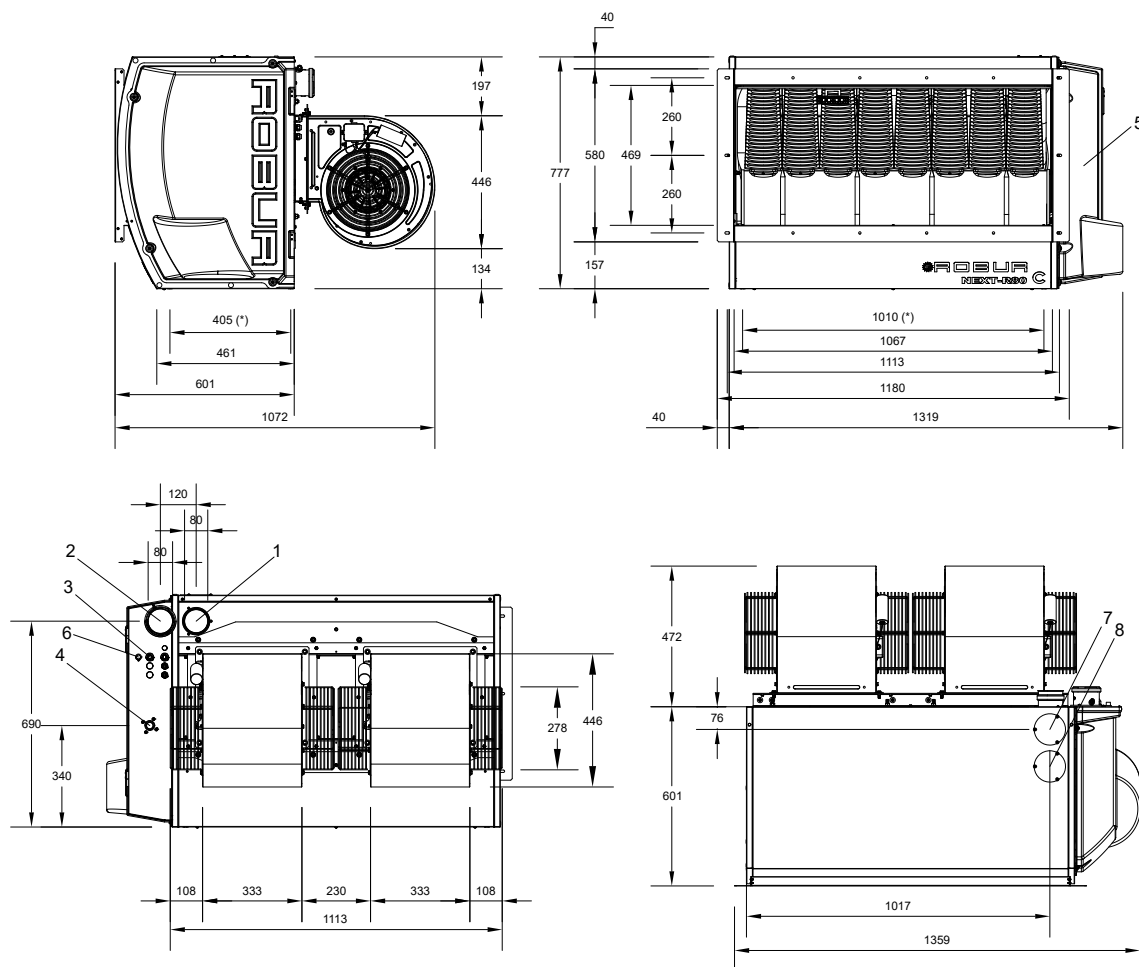
Figura 4.10 Dimensioni unità
