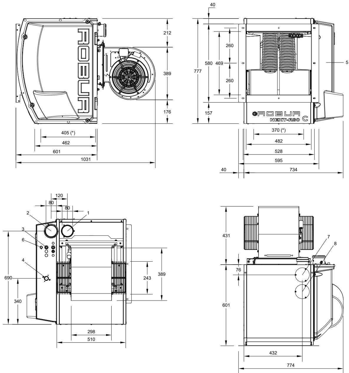
Figura 4.7 Dimensioni unità
