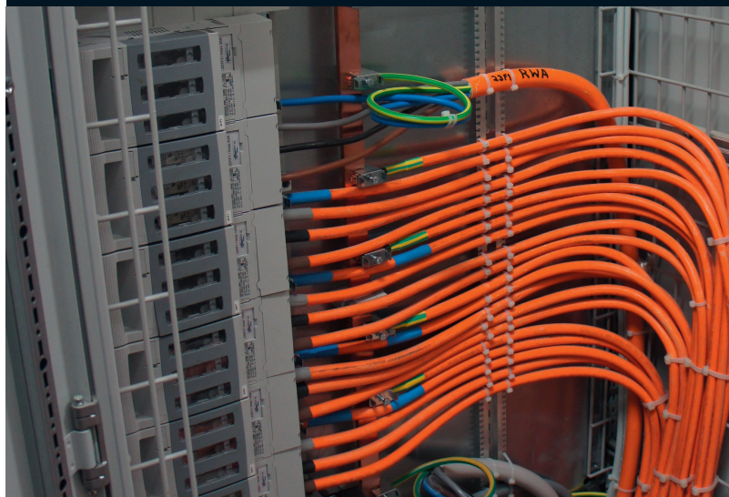
Les interrupteurs sectionneurs HPC ont été montés sur un système RiLine60.
