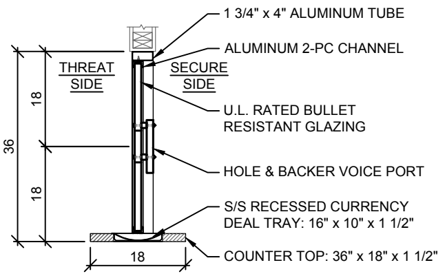
4 SECTION A1
