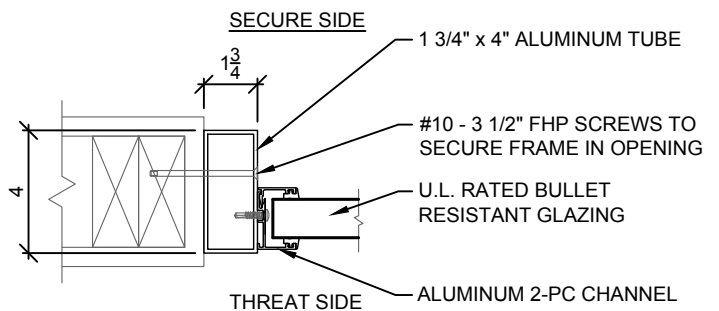
3 DETAIL A1
