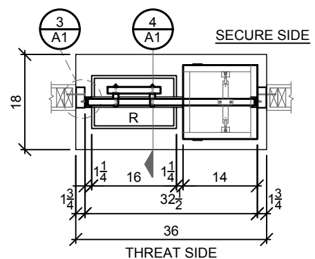
1 PLAN A1
