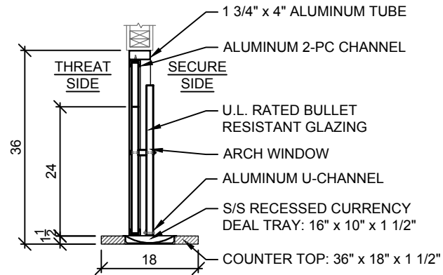
4 SECTION A1
