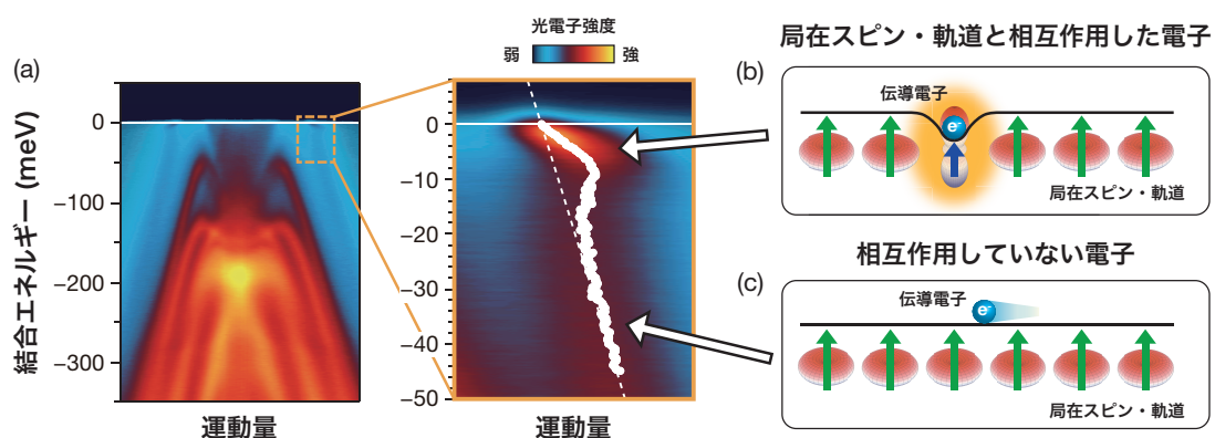
図1 : (a) レーザー光電子分光で観測したセリウム・アンチモン電子構造。相互作用で重くなった伝導電子（準粒子）に対応する電子構造の折れ曲がり観測されました。(b,c) 本研究で明らかにした準粒子の概念図。本来物質中を自由に動き回るはずの伝導電子が、局在スピン・軌道との強い相互作用により質量が増大して動きにくくなります。
