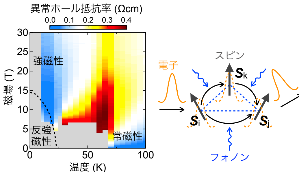
図 3. (左)磁化に比例しない異常ホール抵抗成分の温度磁場相図上の強度。(右)有限のスピнкаイラリティを持つ非共面的なスピン配置におけるホッピング伝導を考慮した異常ホール効果の理論。
