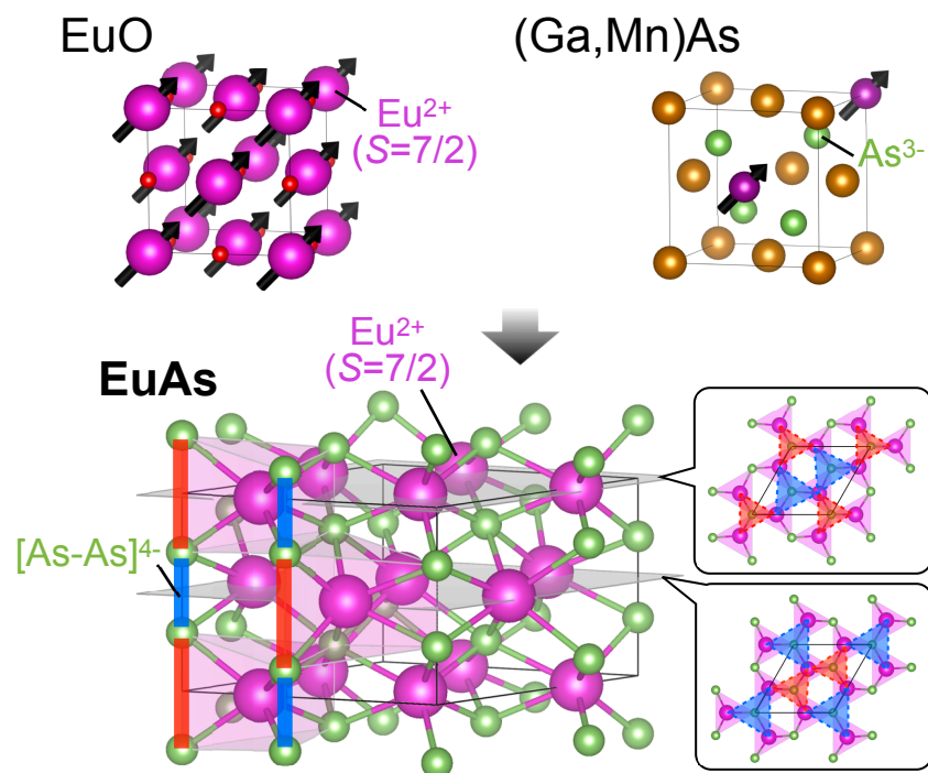
図 1. (上) 代表的な磁性半導体である (Ga, Mn)As と EuO の結晶構造。(下) 本研究で対象とした EuAs の結晶構造。巨大なスピンを持つ Eu 2+ イオンが、異なる大きさの三角形からなる三角格子をなす。
