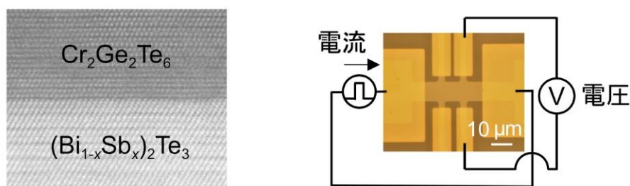
図1 透過型電子顕微鏡による積層構造の断面像と作製したホールバーの光学顕微鏡像
