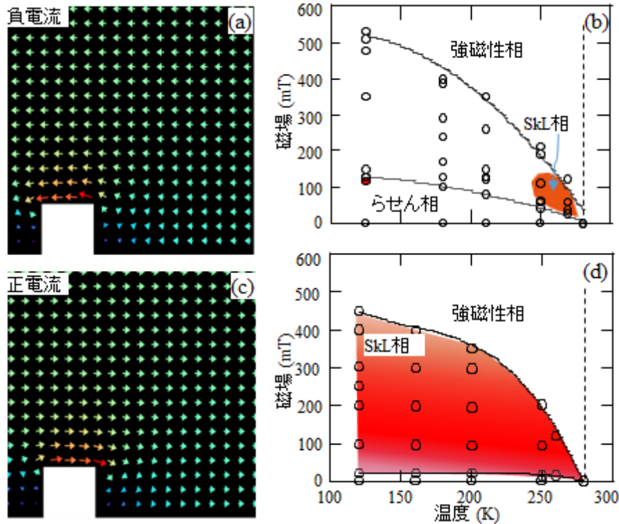
図1 小さな「切り欠き」をつけたデバイスにおける電流密度分布と相図
