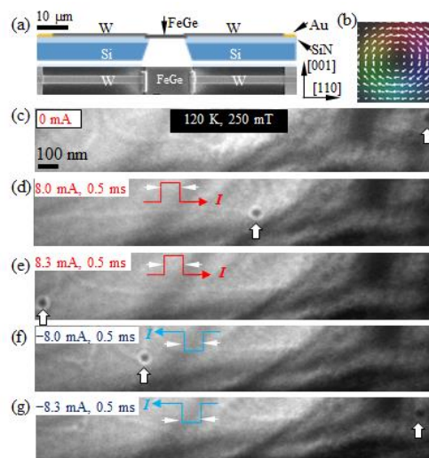
微小電流の正負パルス電流によりスキルミオン（白矢印の黒点）が横方向に移動する様子（c-d）
