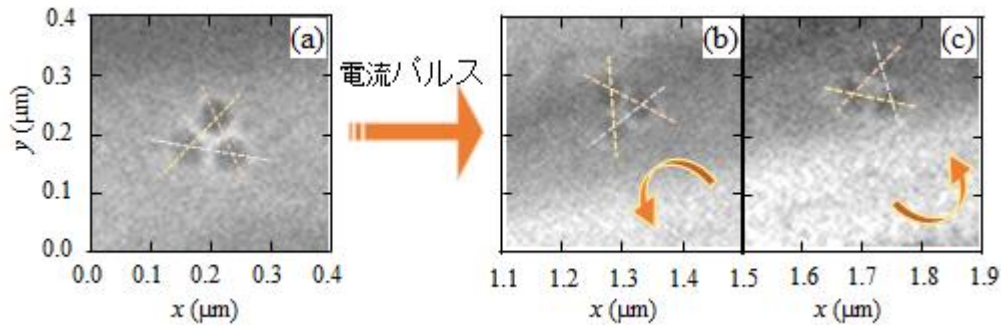
図 4 負電流パルスによるスキルミオンクラスターの回転移動
