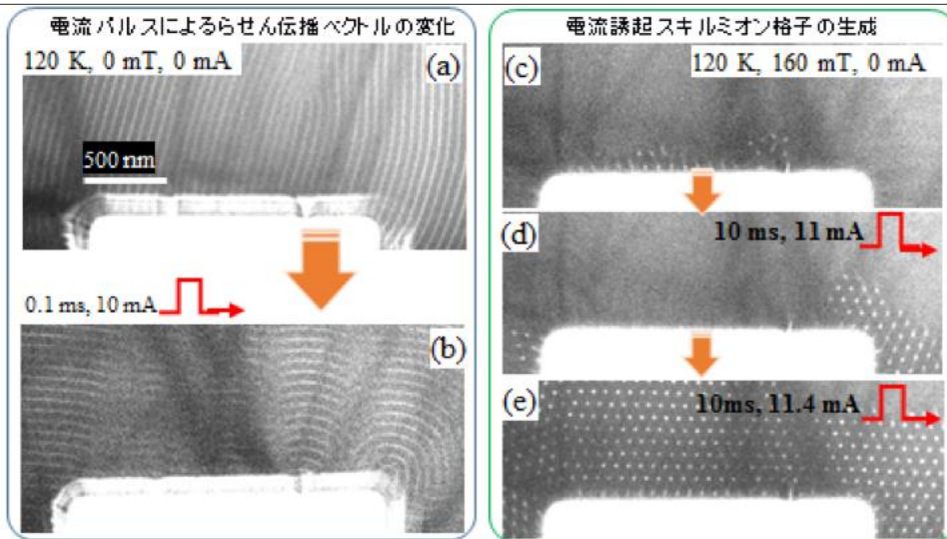
図2 正電流パルスによるらせん磁気構造の伝播方向回転とスキルミオン格子の生成
