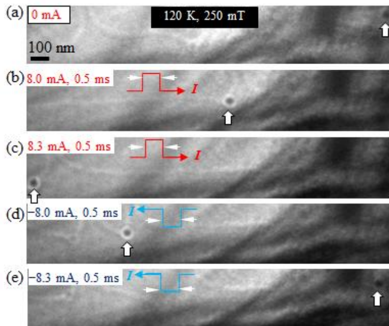
図3 正負パルス電流により単一スキルミオンが横方向に移動する様子
