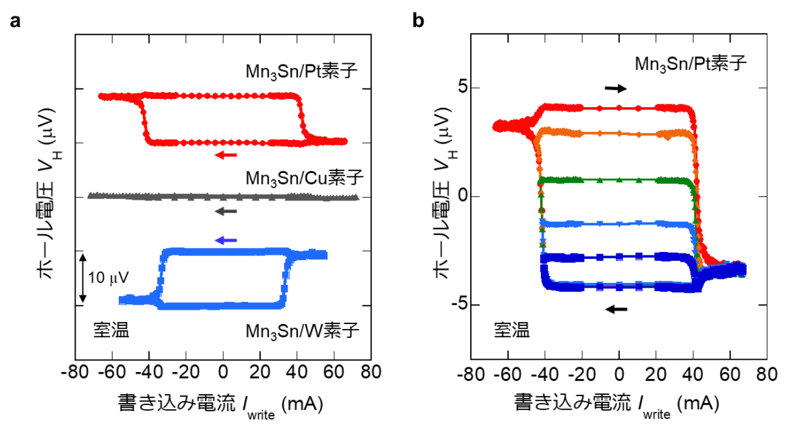
図 4 ワイル反強磁性体 Mn_3Sn /非磁性金属からなる素子でのホール電圧の電流反転 (a)ワイル反強磁性体 Mn_3Sn と白金 (Pt)、銅 (Cu)、タングステン (W) との積層膜を用いた素子における、ホール電圧の書き込み電流依存性。大きなスピンの発生が期待できる Pt もしくは W からなる素子において、ホール電圧の反転が確認できます。Mn 3 Sn /W 素子ではホール
