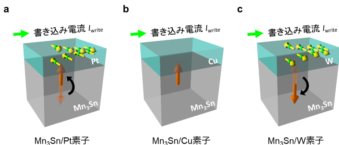
図5 ワイル反強磁性体 \text{Mn}_3\text{Sn} /非磁性金属の素子でのスピンの流による仮想磁場反転の概要図 白金 (Pt (a)) やタングステン (W (c)) では、電流を流すことで黄色矢印に偏極した大きなスピンの流が生じます。このスピンの流によりワイル反強磁性体 \text{Mn}_3\text{Sn} の反強磁性秩序・ワイル点およびその仮想磁場 (オレンジ矢印) が反転し、仮想磁場由来の異常ホール効果の反転が起こります。一方で、銅 (Cu (b)) では、ほとんどスピンの流が生じないため、異常ホール効果の反転は起きません。従って図 4a の電流によるホール電圧の反転は、非磁性金属で生成されたスピンの流の効果と考えられます。
