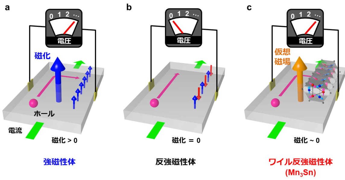
図 3 強磁性体と反強磁性体、ワイル反強磁性体 Mn_3Sn における異常ホール効果 (a) 大きな磁化を持つ強磁性体では異常ホール効果が現れます。一般に、磁化の大きさに比例して異常ホール効果は大きくなります。(b)反強磁性体では磁化が0、もしくは、非常に小さいため、異常ホール効果の測定は困難です。(c)ワイル反強磁性体 Mn_3Sn では、ワイル点が創出する仮想磁場の効果により、磁化が非常に小さくても、強磁性体に匹敵するほど大きな異常ホール効果が現れます。
