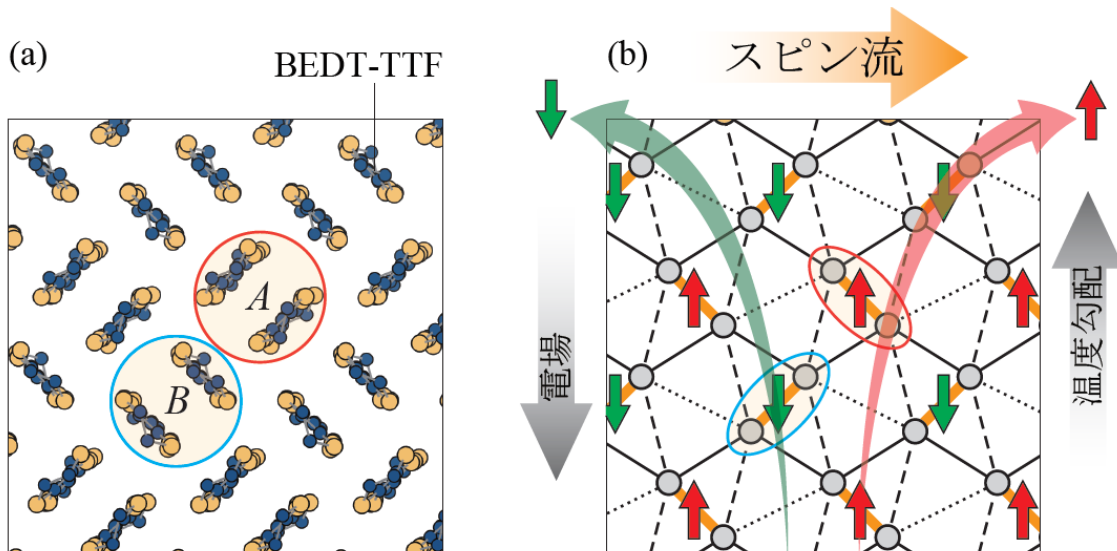
図 1 : (a) \kappa -(BEDT-TTF) 2 Cu[N(CN) 2 ]Cuの分子配列。A、Bはそれぞれ分子ペアを表す。 (b) 反強磁性状態の電子スピン配列とスピン流生成の様子。
