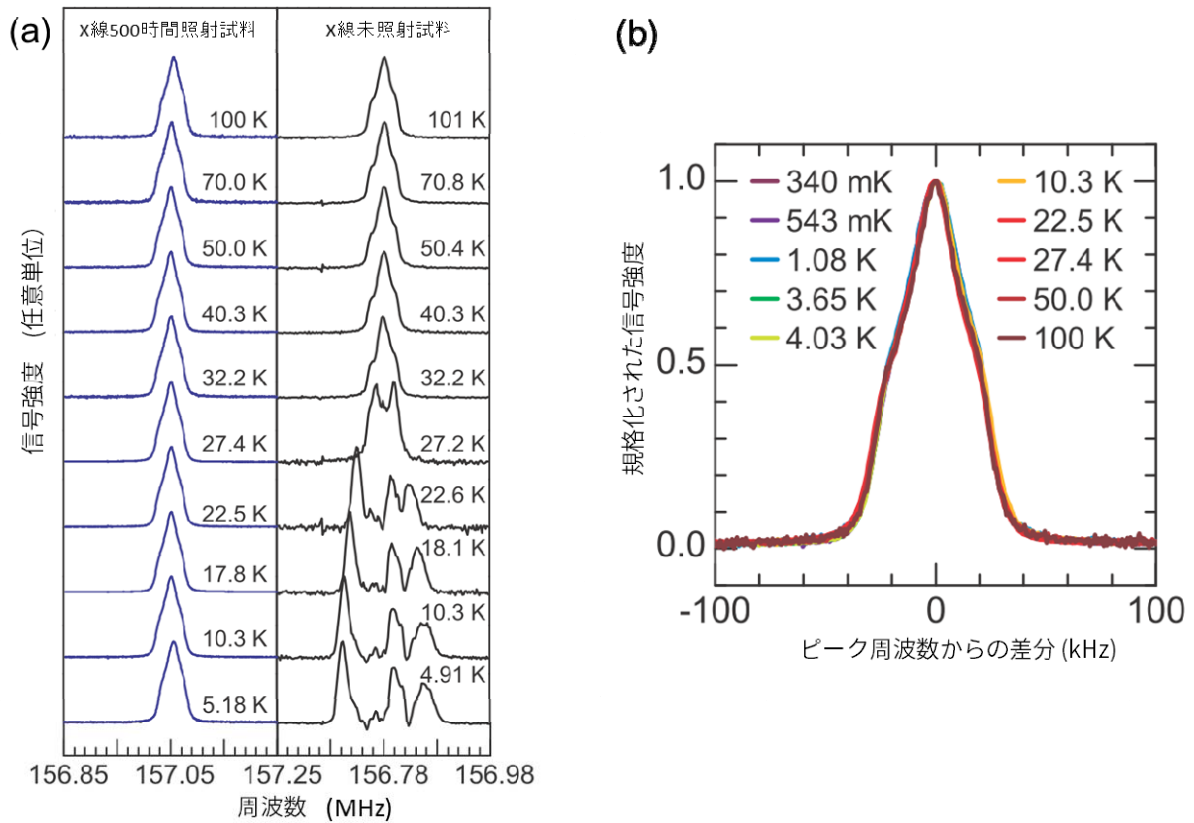
図2 \kappa -(ET) 2 Cu[N(CN) 2 ]Cl の核磁気共鳴スペクトル
