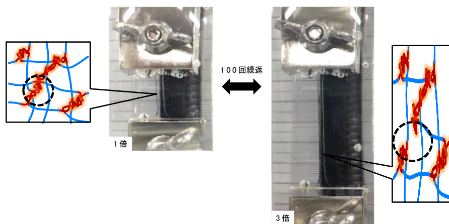
図2 引張耐久性試験におけるゲルの網目構造の変化。
