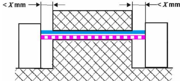
그림 0.6 — 좁은 홈의 비접착 접합부
