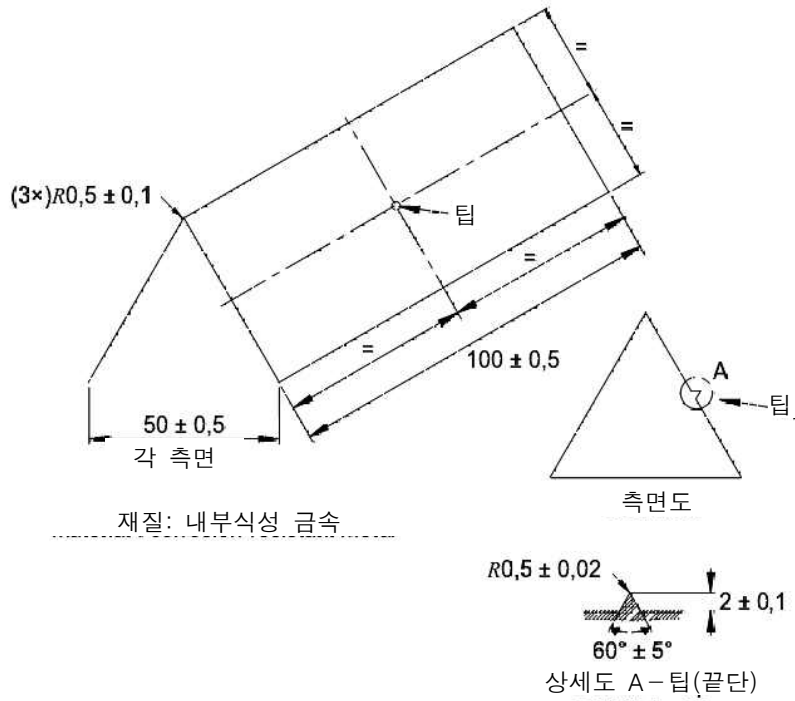
그림 21 — 맨드릴
