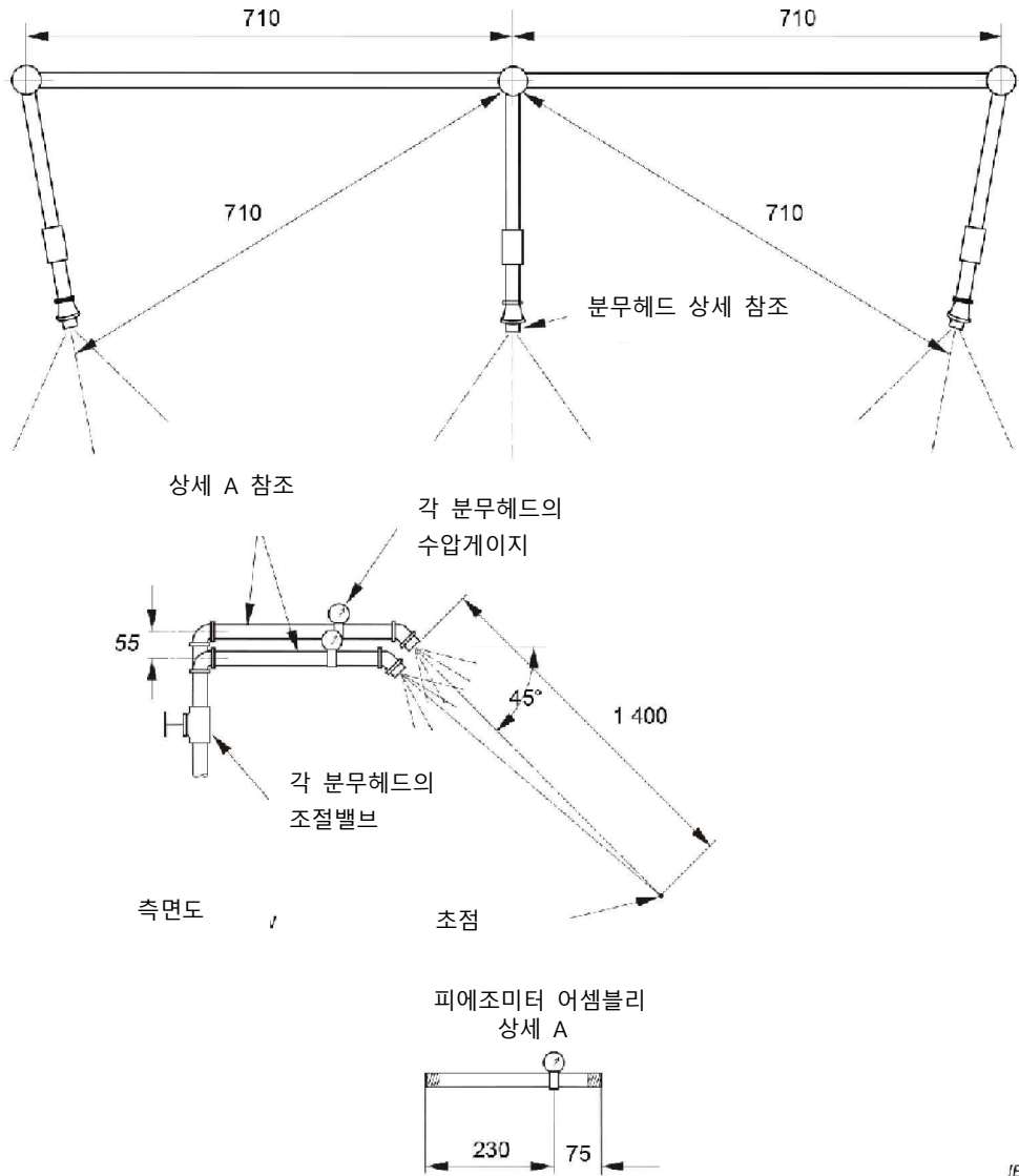
그림 Y.2 - 물 분무 시험 분무 헤드 파이핑
