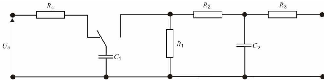
그림 D.1 — 1.2/50 \mu\text{s} 와 10/700 \mu\text{s} 전압 임펄스 발생기
