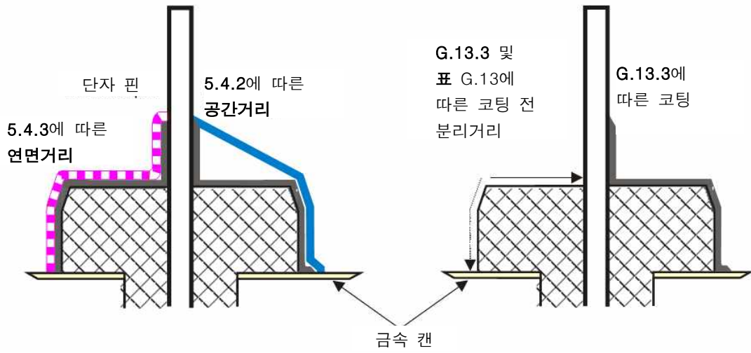
그림 0.11 — 단자 주위 코팅
